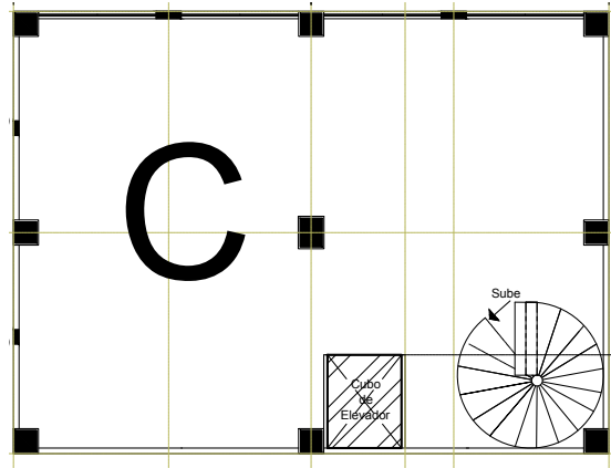
PLANTA TIPO
