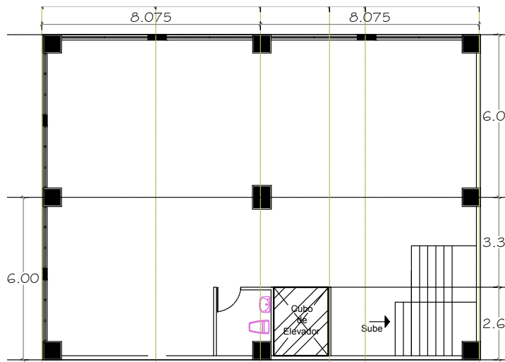
PLANTA TIPO
