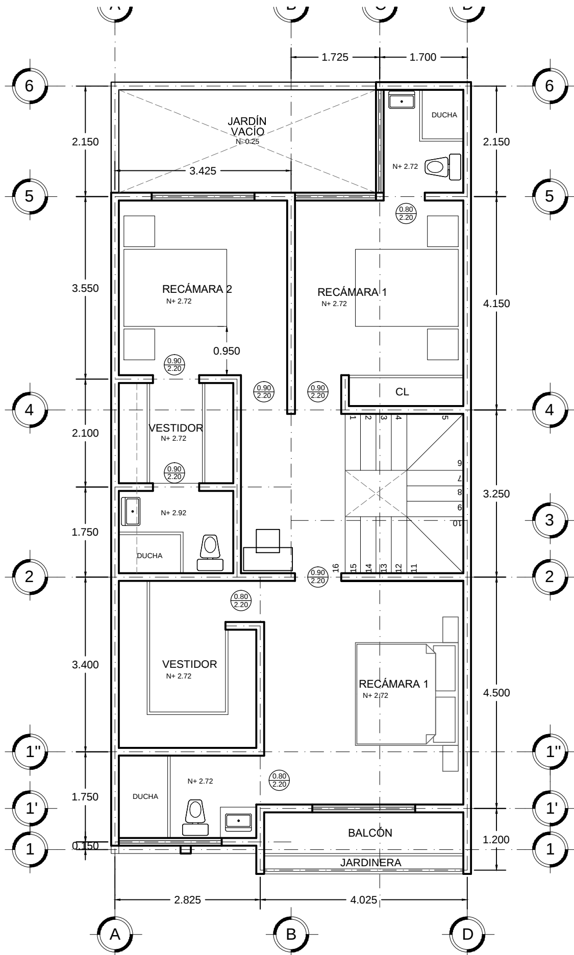
PLANTA ALTA CALLE
