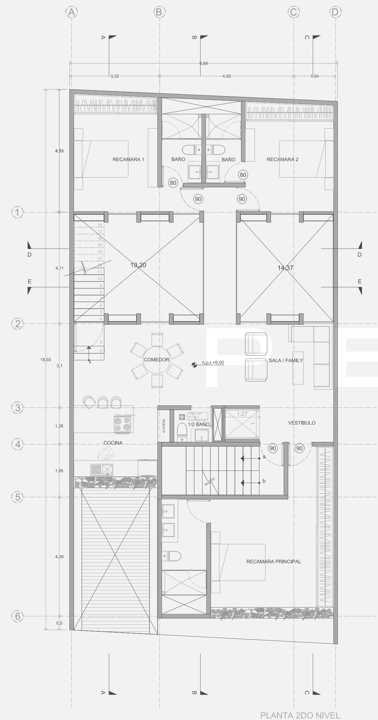
PLANTA 2DO NIVEL
