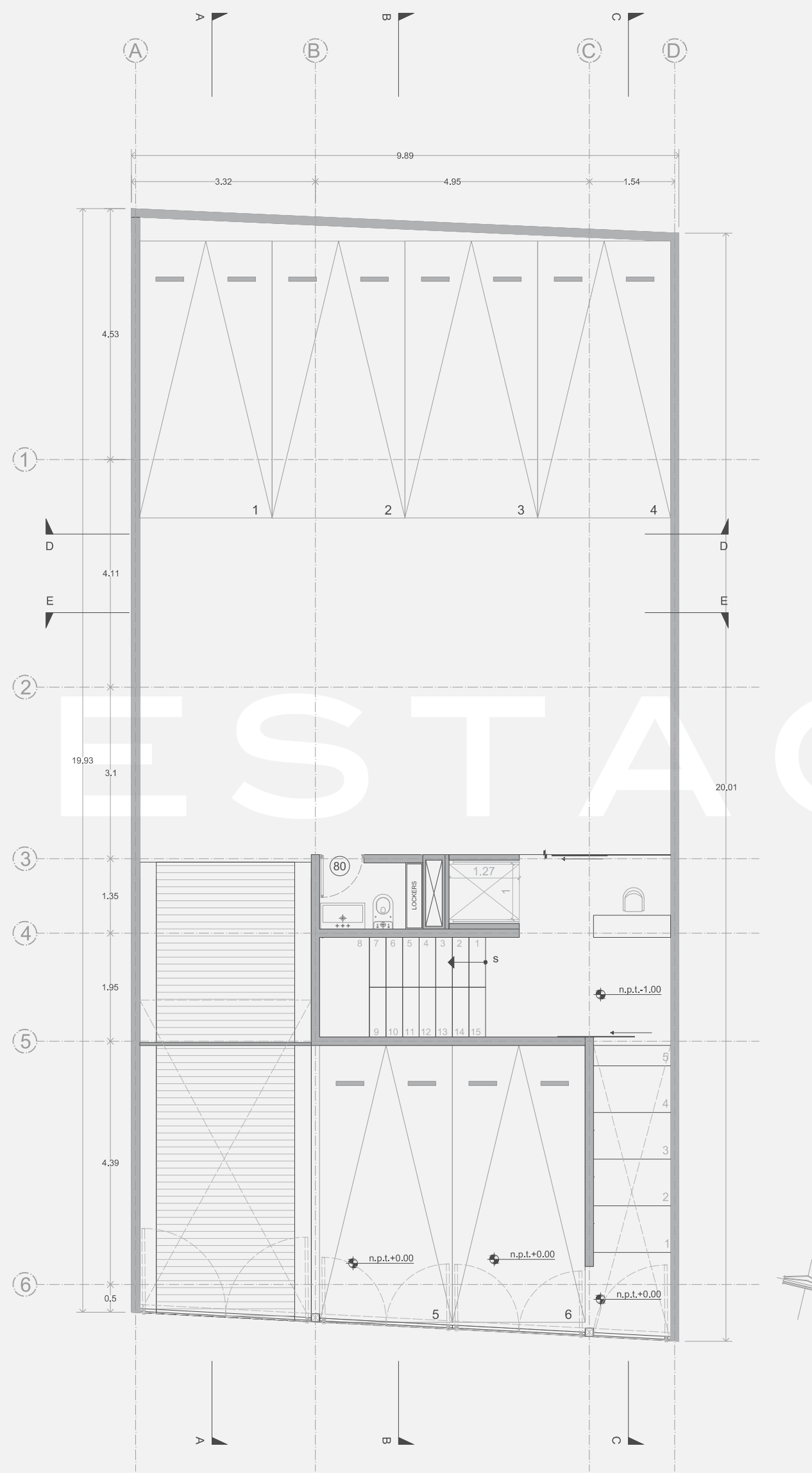
PLANTA ESTACIONAMIENTO
