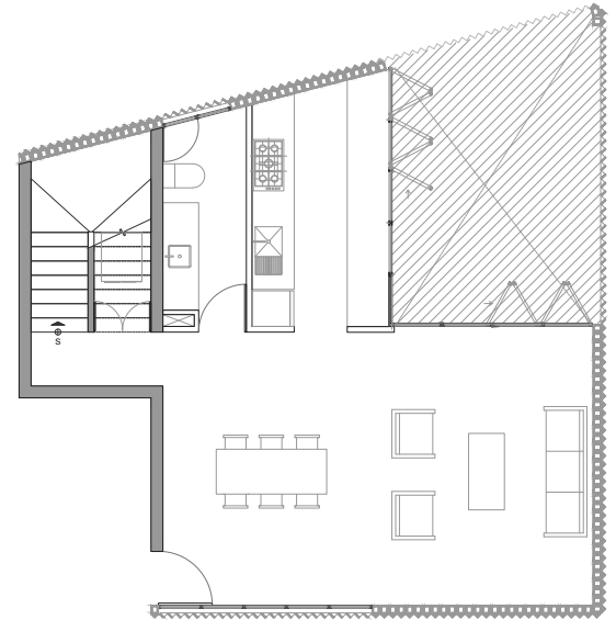
planta nivel 2
