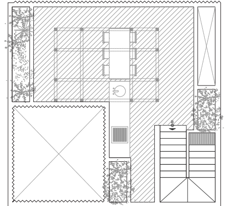
planta azotea
