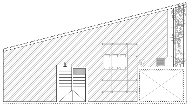
planta azotea
