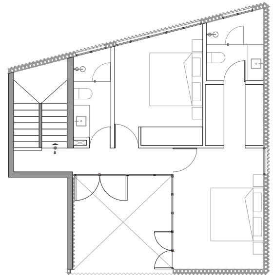
planta nivel 1
