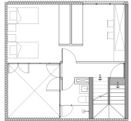
planta nivel 3
