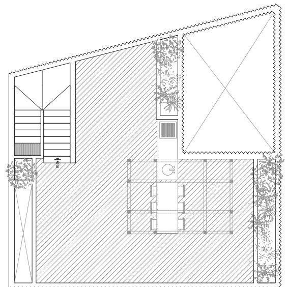
planta azotea
