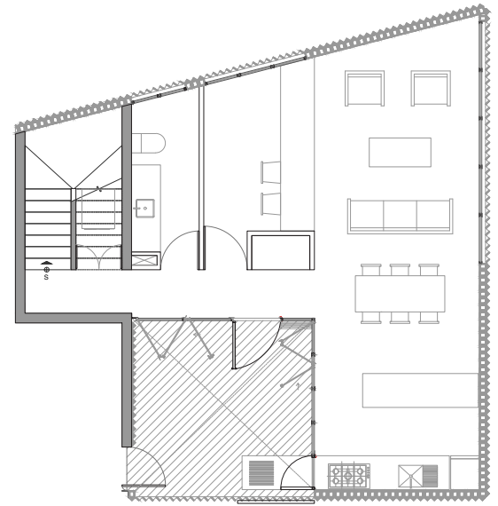
planta baja
