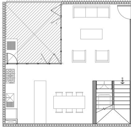
planta baja
