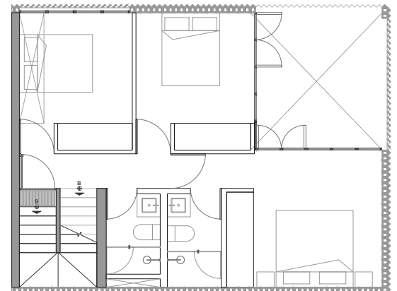
planta nivel 3
