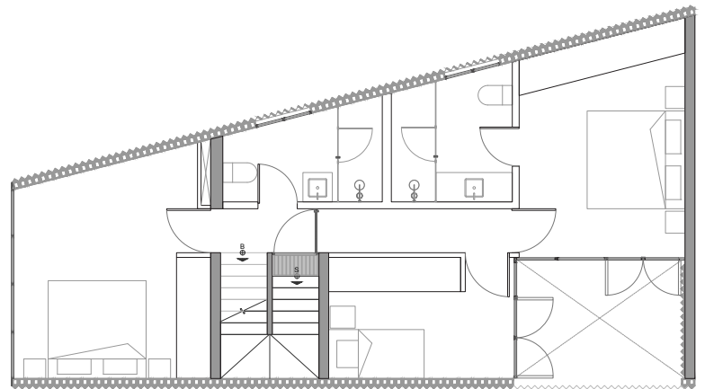
planta nivel 3
