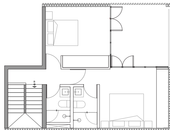
planta nivel 1
