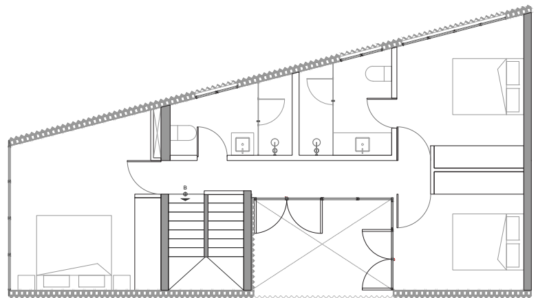
planta nivel 1
