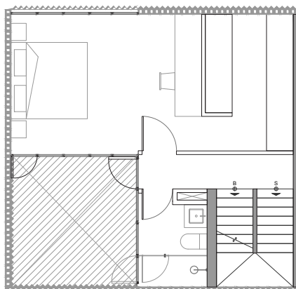
planta nivel 2
