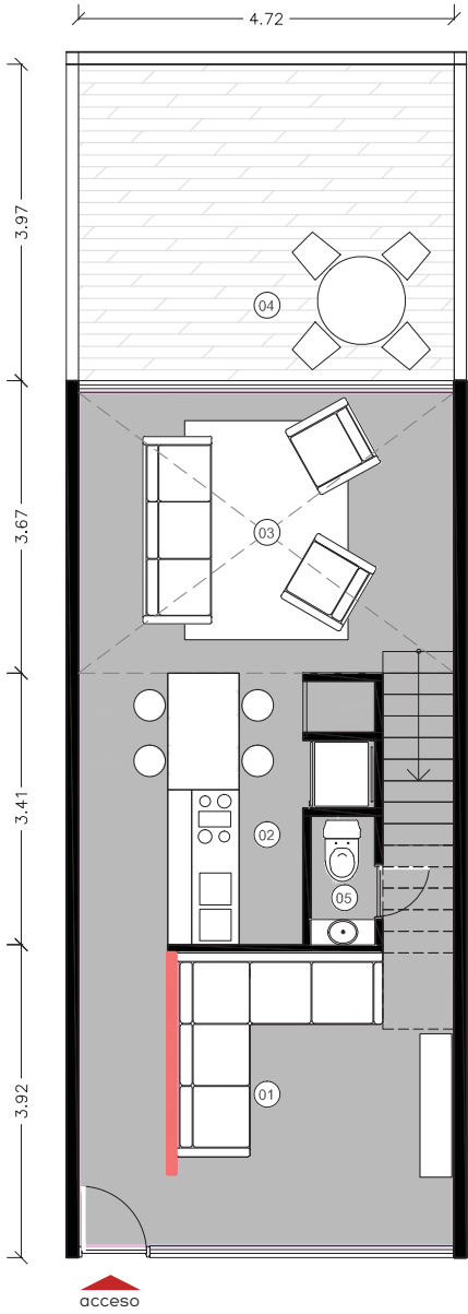
Planta Baja | N + 1.20
