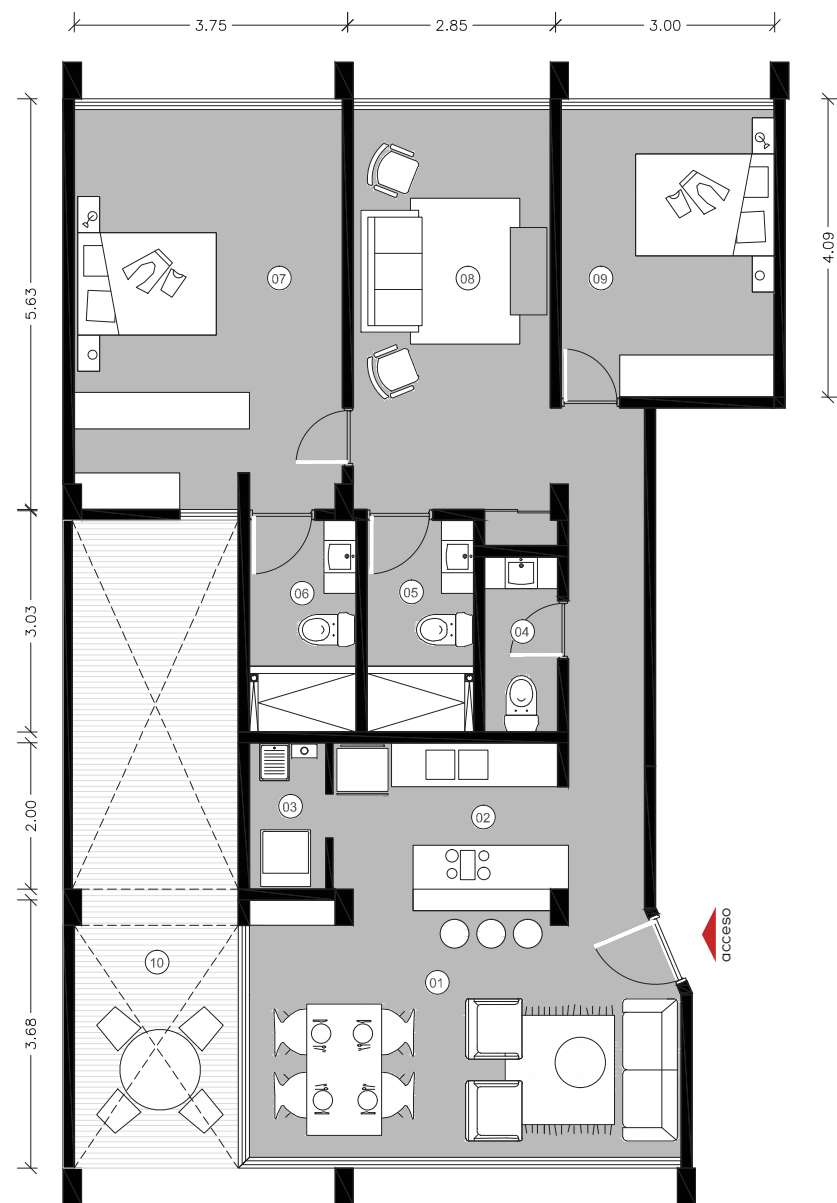
Planta Baja | N + 3.28
