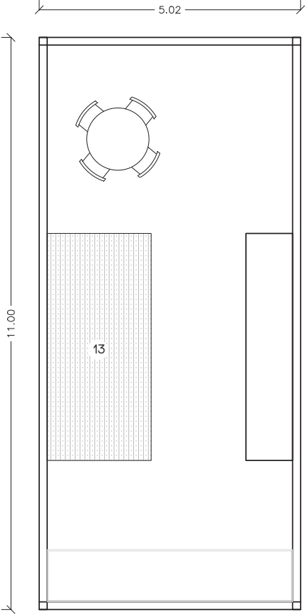
Planta Alta | N + 12.00
