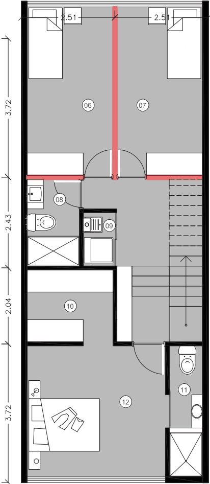
Planta Alta | N + 5.16
