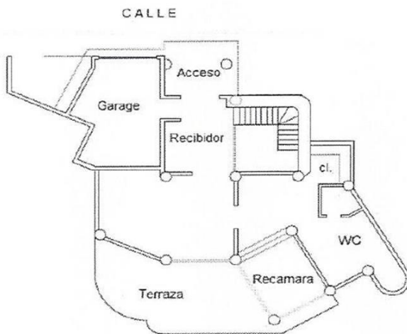
PLANTA ALTA
