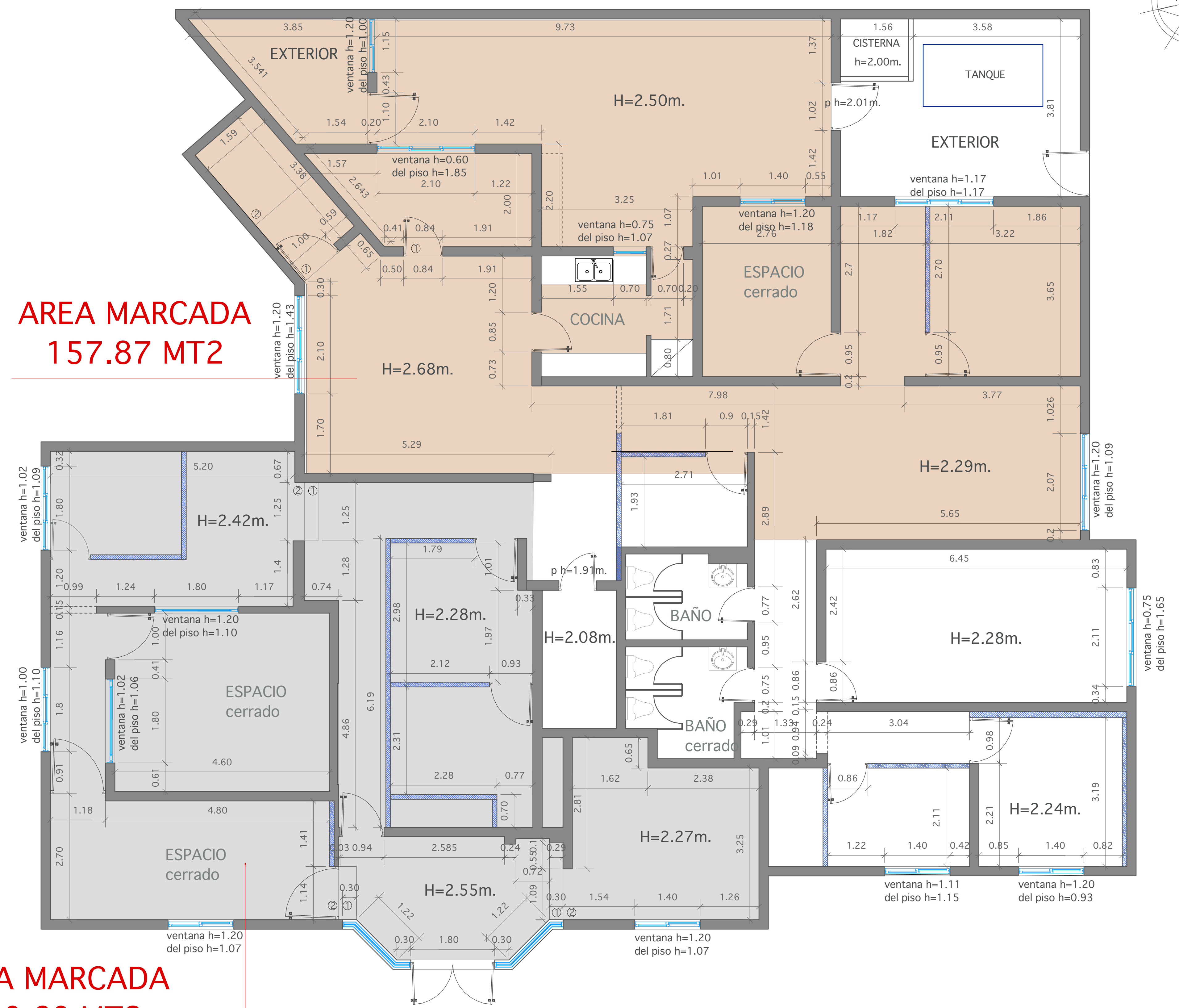
2 A 1 LEVANTAMIENTO PLANTA ARQUITECTONICA COMERCIAL-OFICINA ESC.: 1:50
