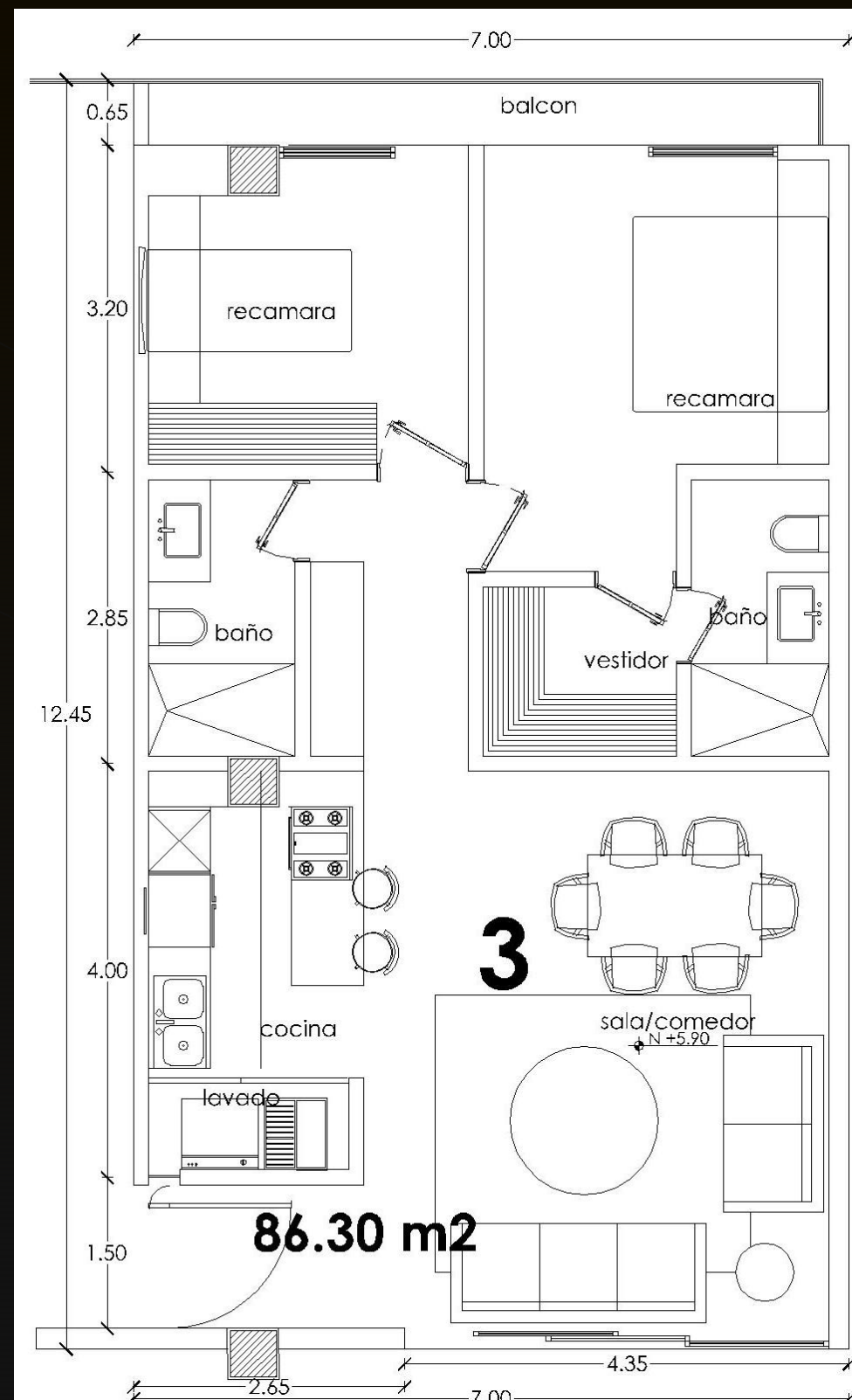
DEPARTAMENTO TIPO 3
