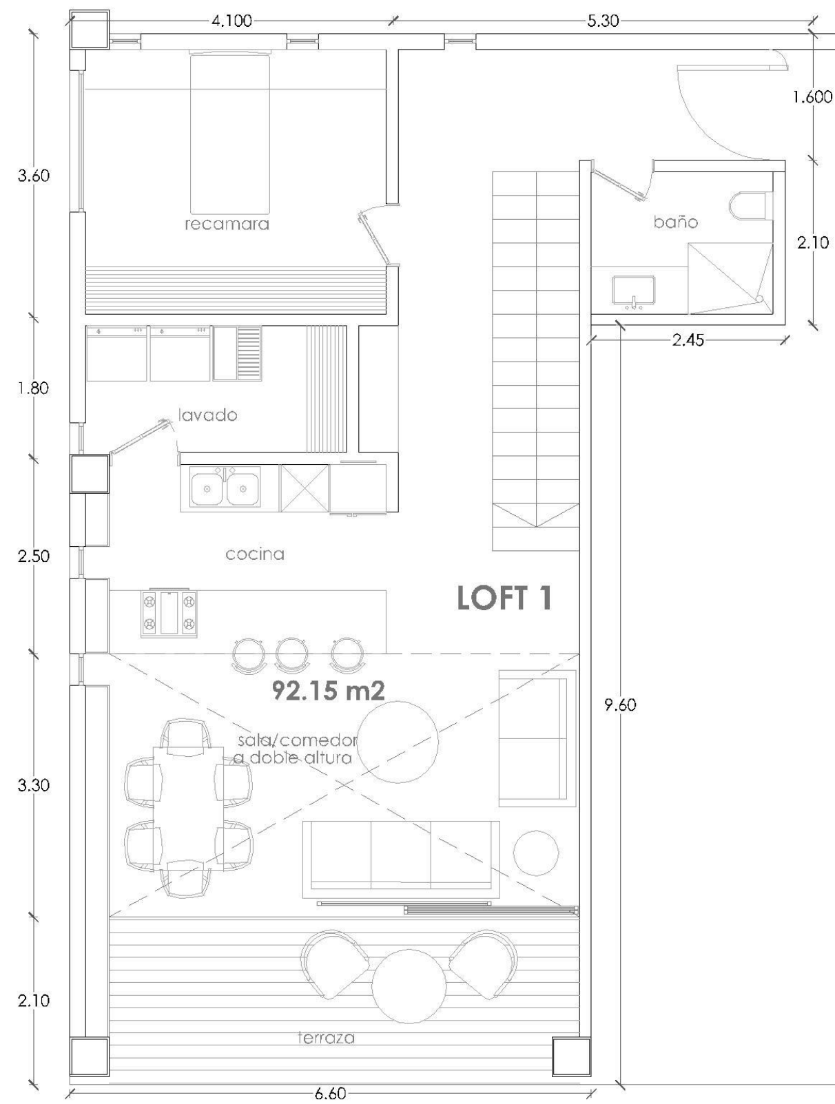
PLANTA BAJA
