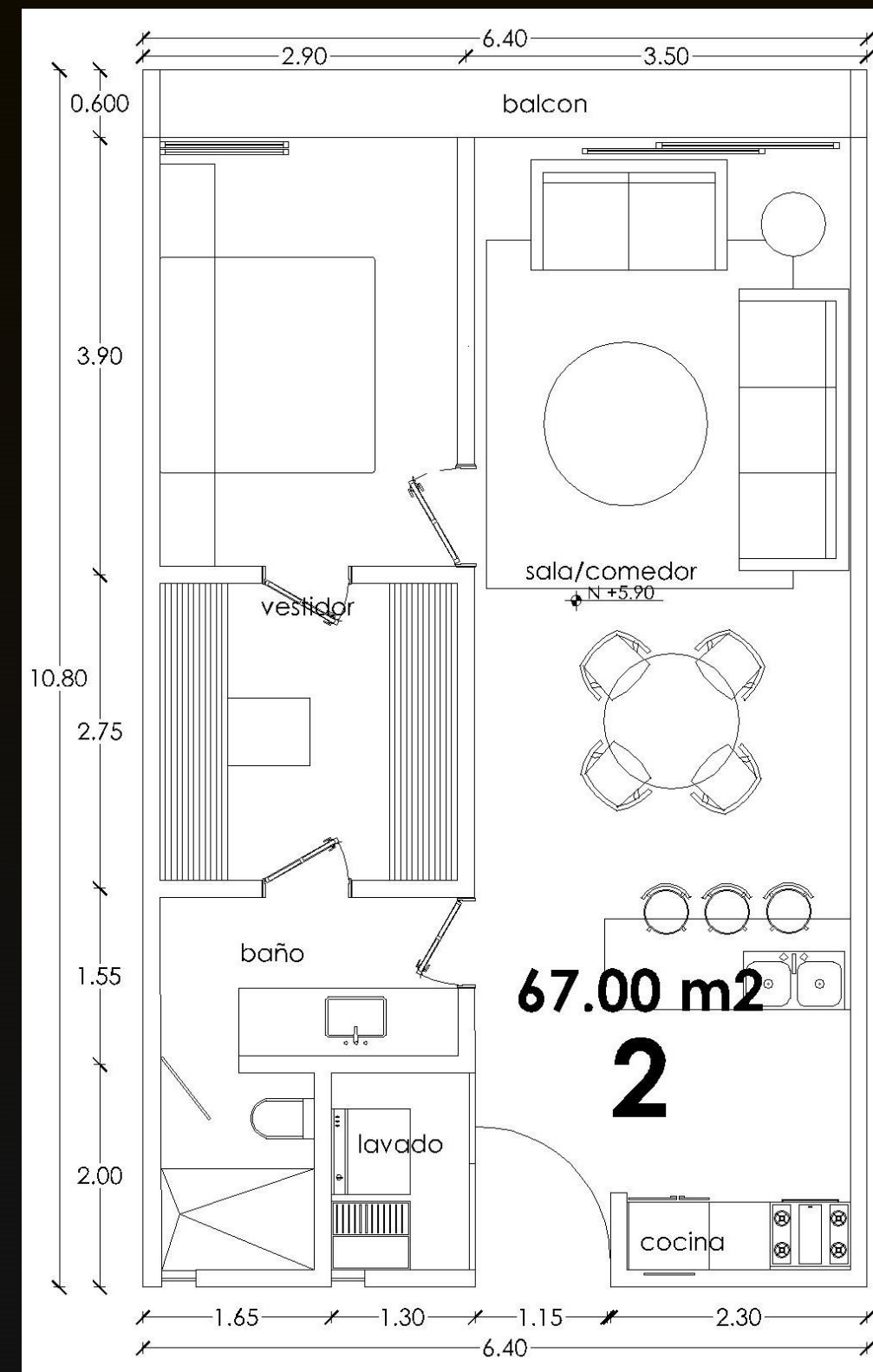
DEPARTAMENTO TIPO 2
