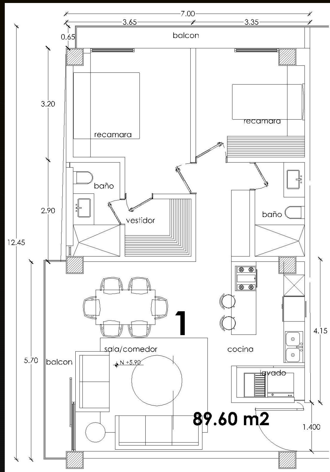
DEPARTAMENTO TIPO 1
