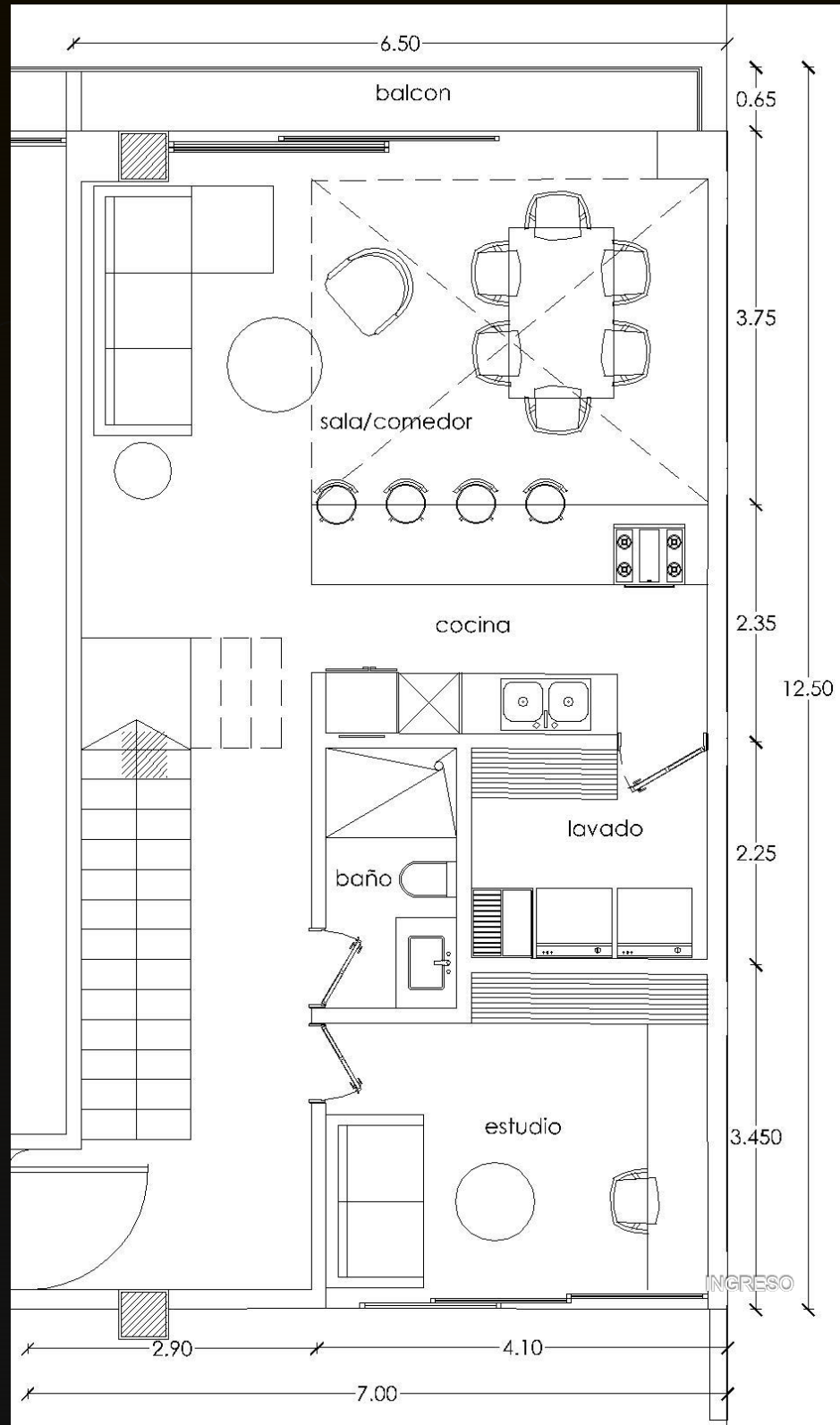
PLANTA BAJA
