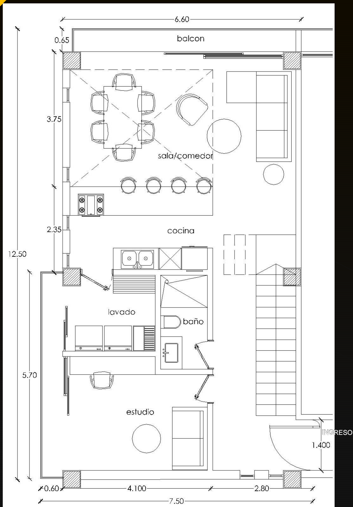
PLANTA BAJA
