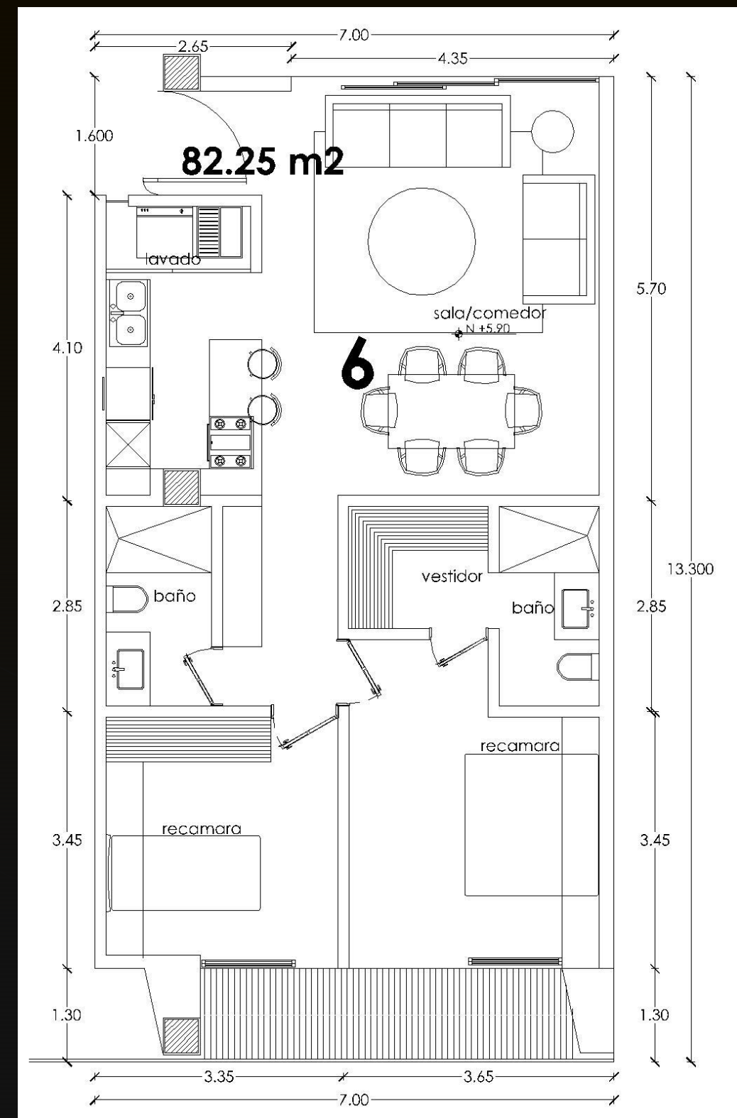
DEPARTAMENTO TIPO 6
