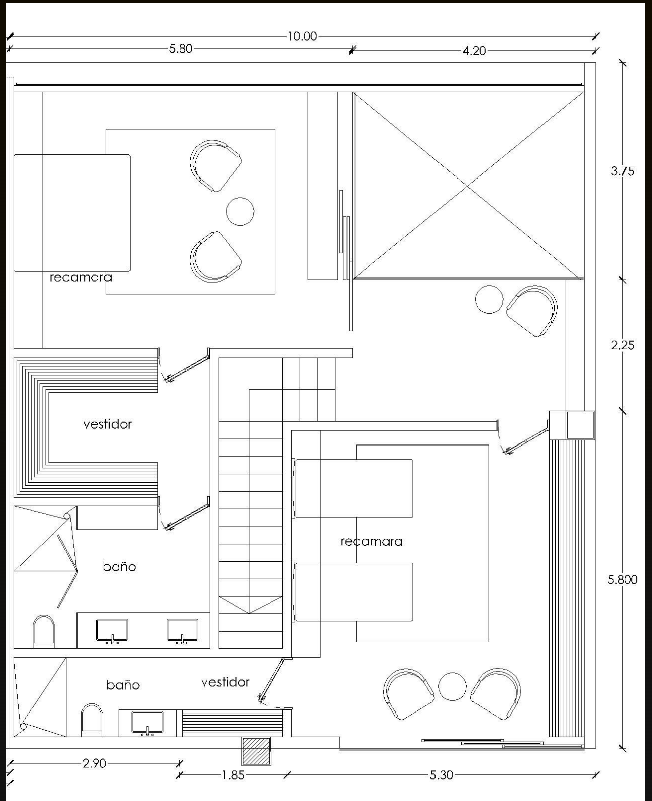
PLANTA ALTA
