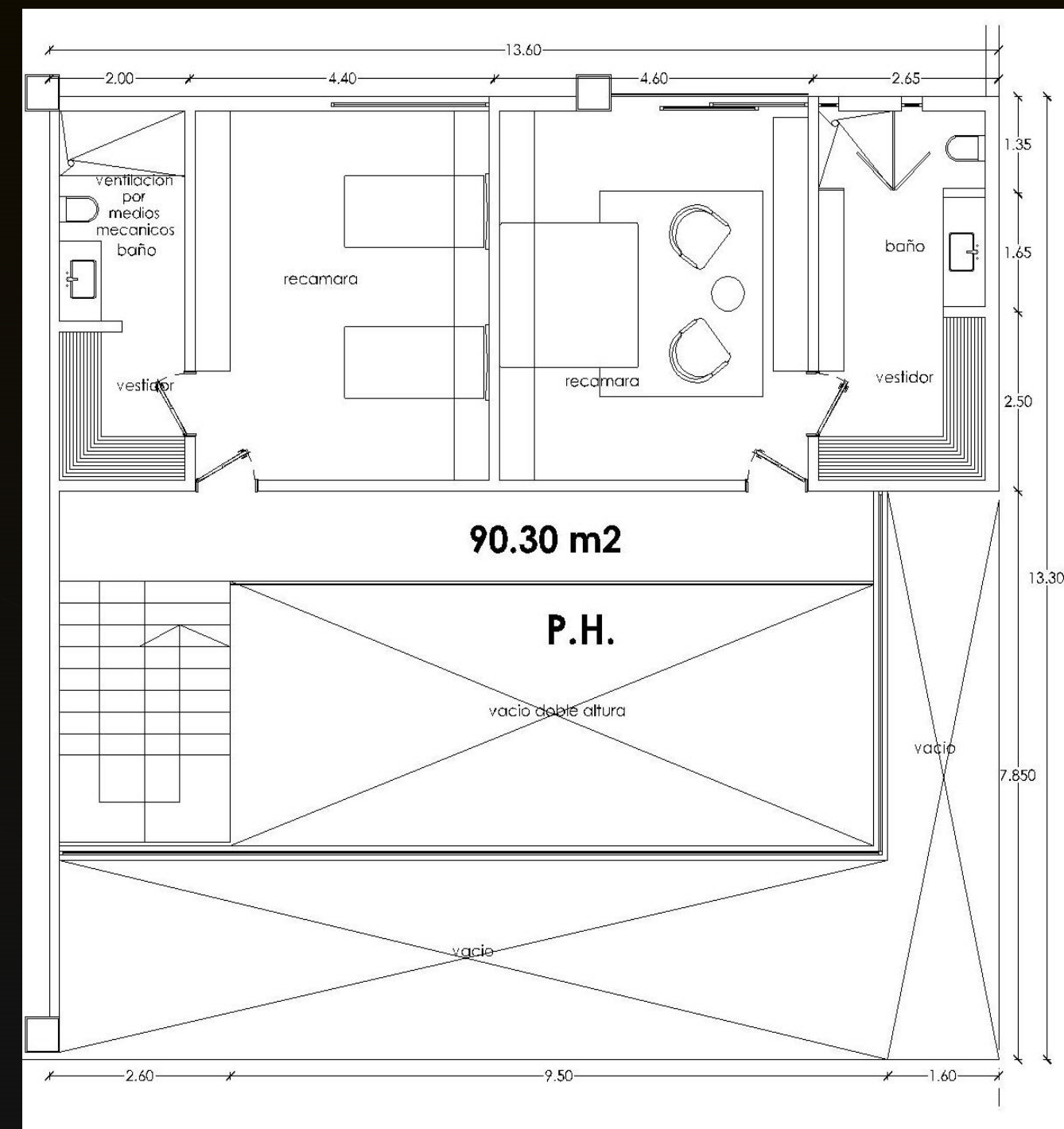
PLANTA ALTA
