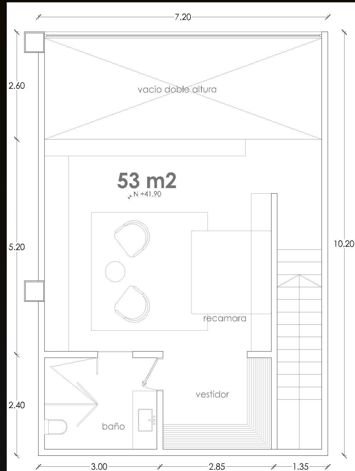
PLANTA ALTA
