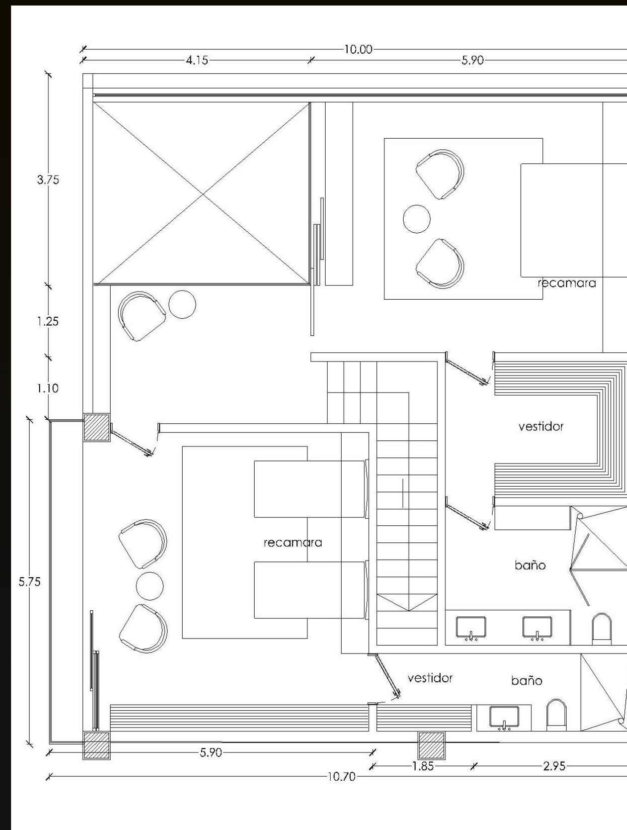
PLANTA ALTA
