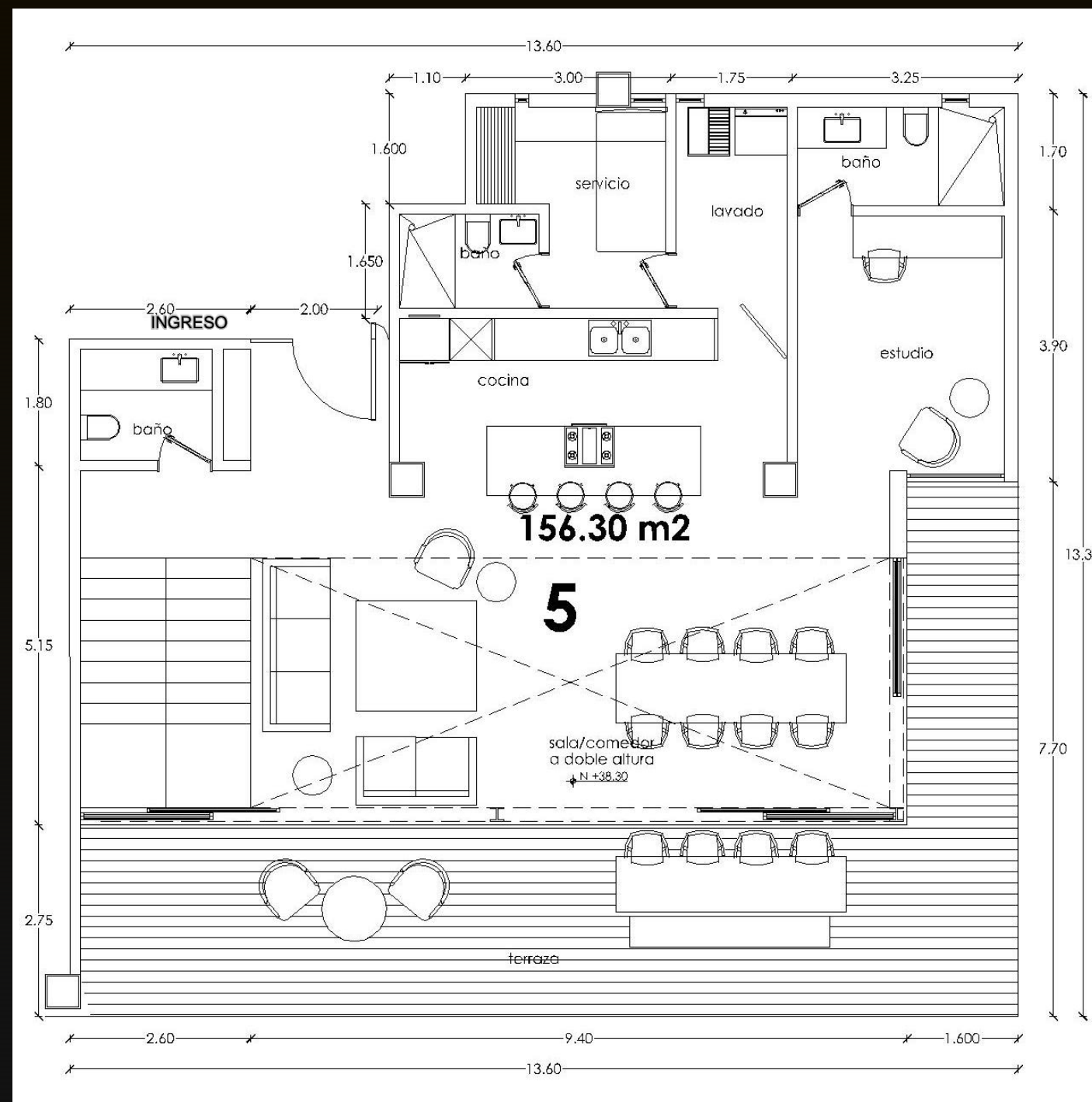
PLANTA BAJA
