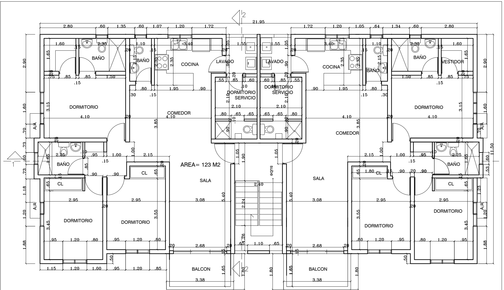
2DA , 3RA Y 4TA. PLANTA ARQUITECTONICA DIMENSIONADABLOQUE B
