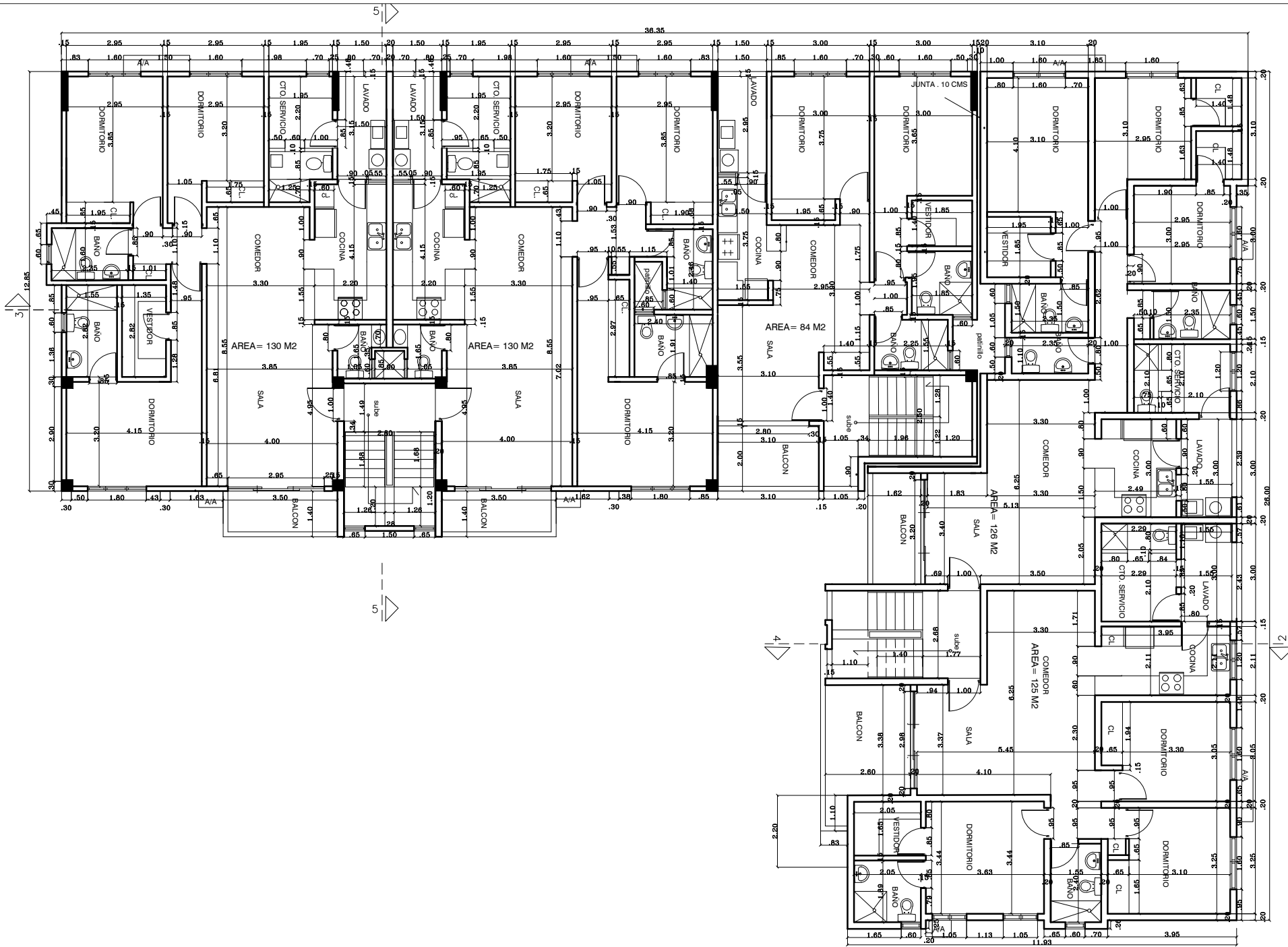
2DA , 3RA Y 4TA. PLANTA ARQUITECTONICA DIMENSIONADA BLOQUE A
