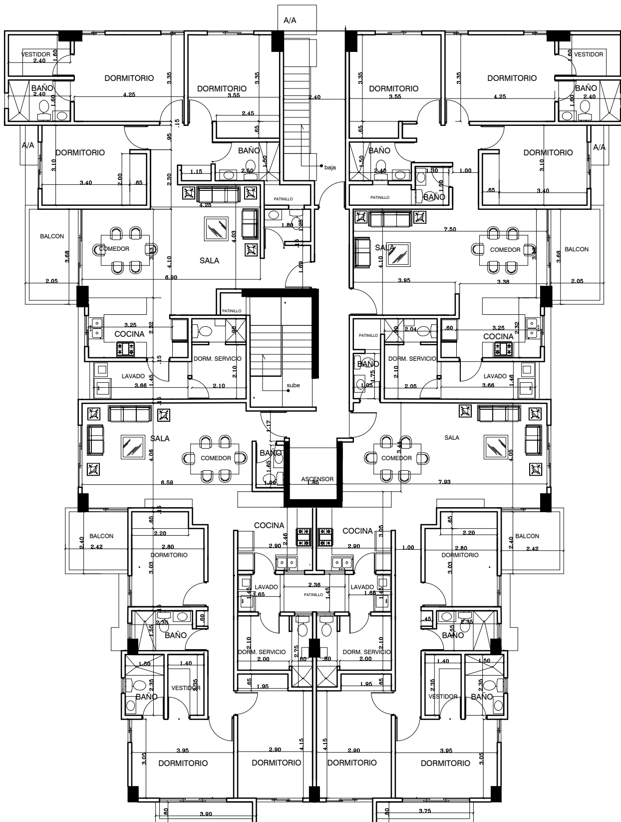
PLANTA ARQUITECTONICA DINENCIONADA 3RA. HASTA 7MA PLANTA
