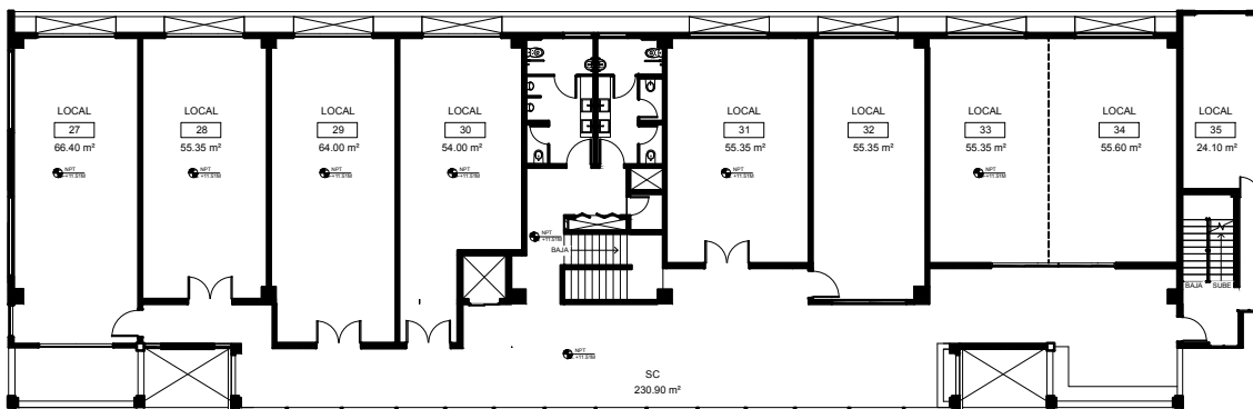
PLANTA CUARTO NIVEL EDIFICIO OFICINA
