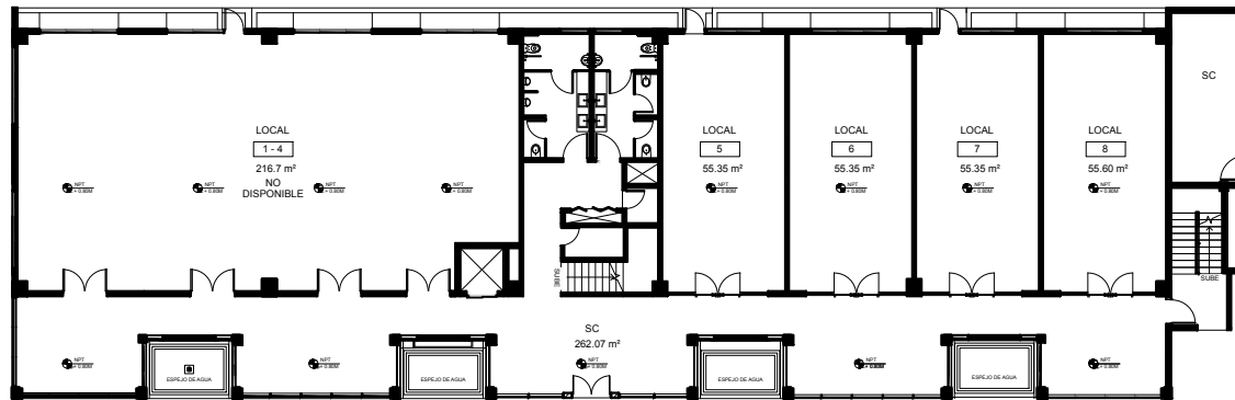
PLANTA PRIMER NIVEL EDIFICIO OFICINA
