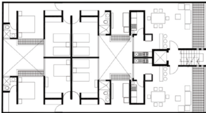
PLANTA TIPO
