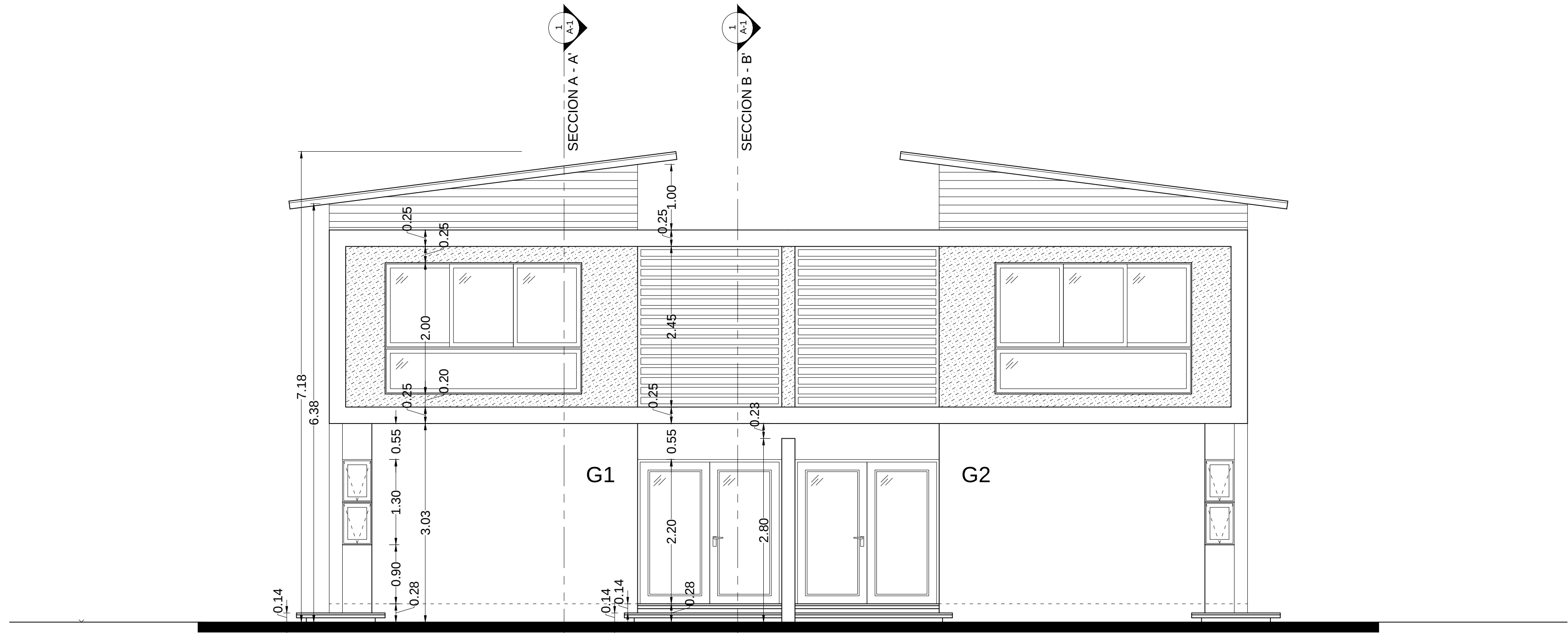
1 A-2 ELEVACION FRONTAL ESCALA 1:50
