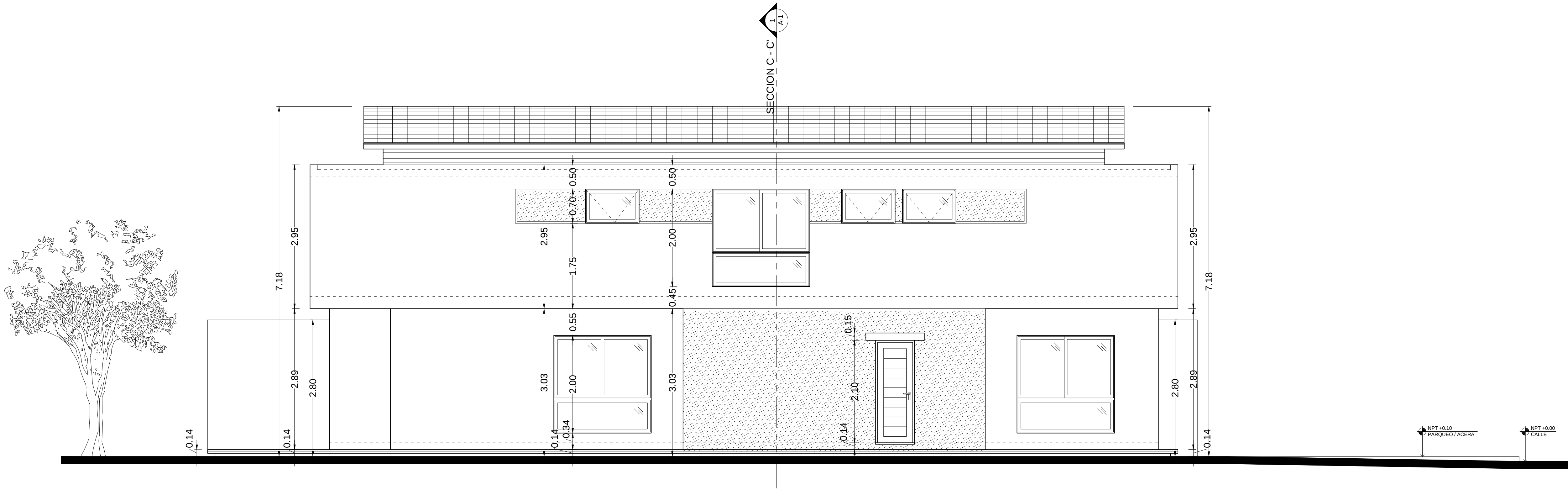
1 A-2 ELEVACION LATERAL IZQUIERDO ESCALA 1:50
