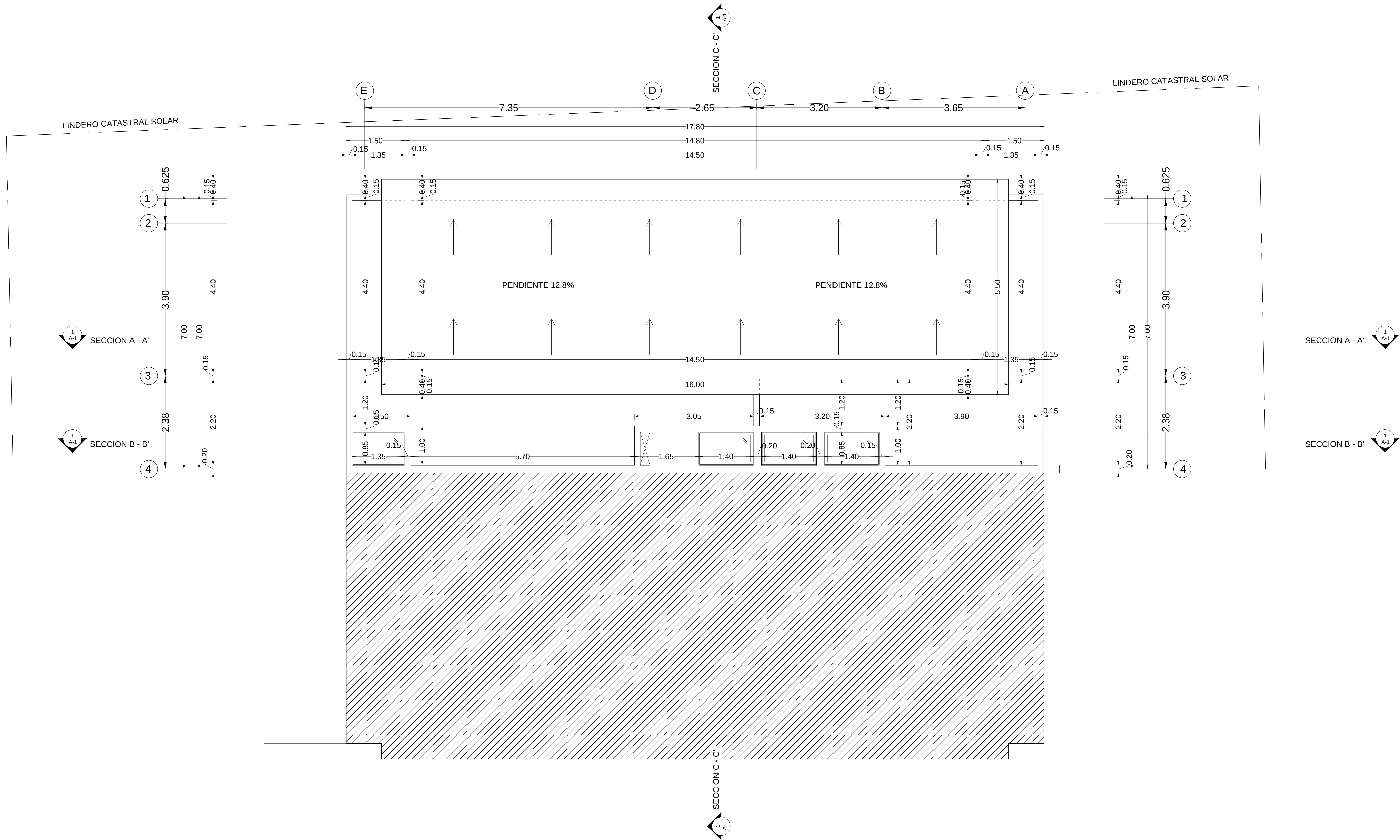
1 A-2 PLANTA DIMENSIONADA DE TECHO ESCALA 1:50
