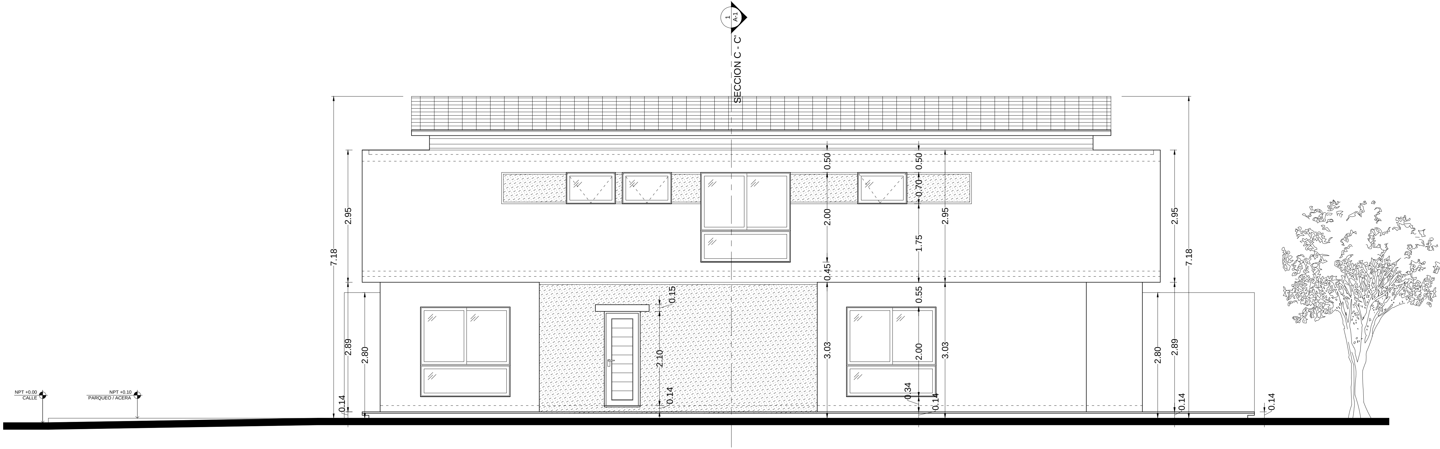
1 A-2 ELEVACION LATERAL DERECHO ESCALA 1:50
