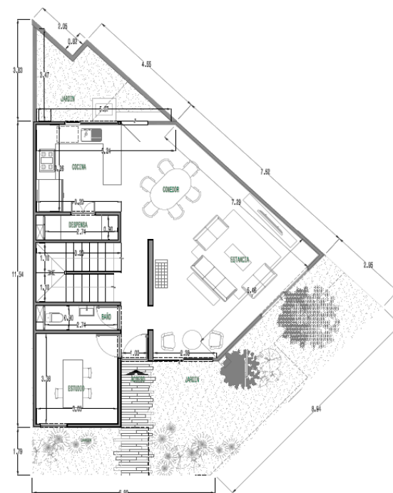
PLANTA BAJA
