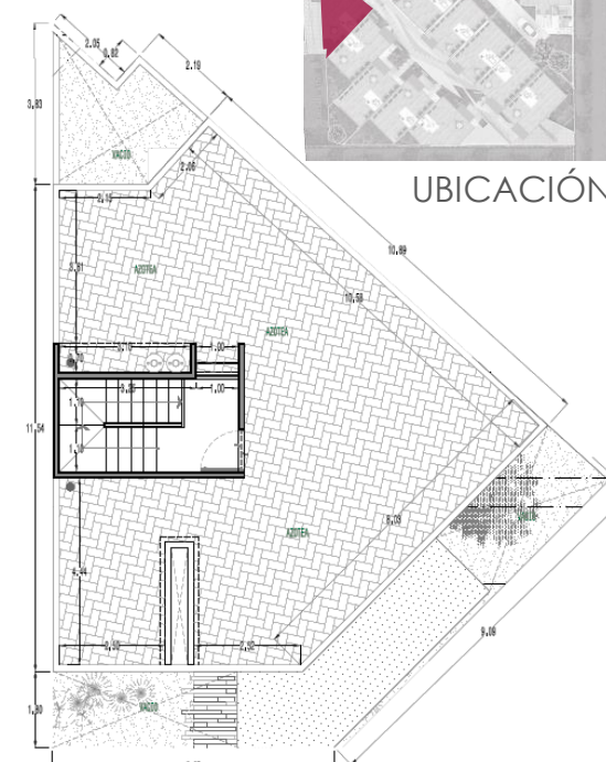
PLANTA AZOTEA
