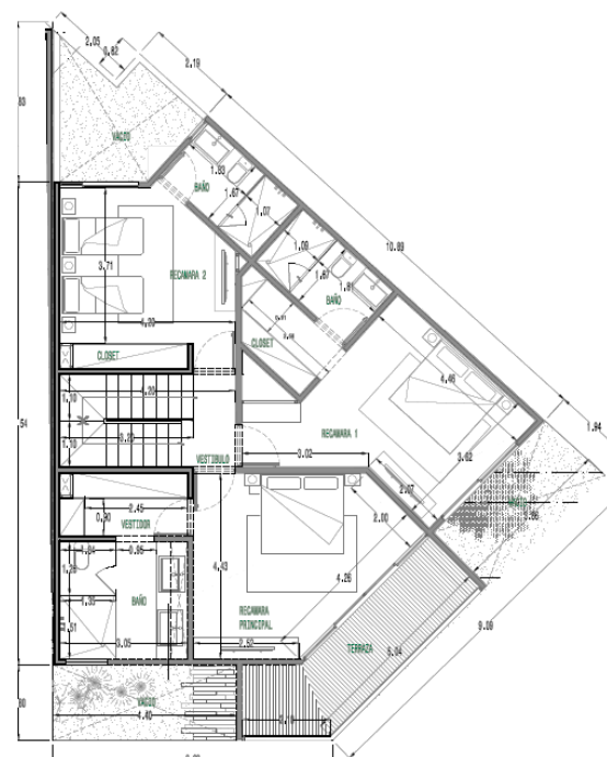
PLANTA ALTA
