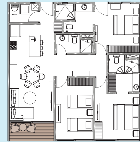
Family Villa 120 m 2 Torre A y C / Niveles 1, 2 y 3 HABITACIÓN LOCK-OFF
