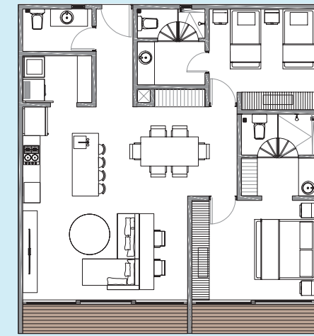
Villa 116 m 2 Torre A y C / Niveles 1, 2 y 3
