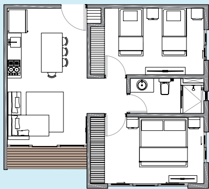
Deluxe 65 m 2 2 recámaras, 1 baño, cocina, comedor y sala con balcón Torre B / Niveles 1, 2, 3 y 4
