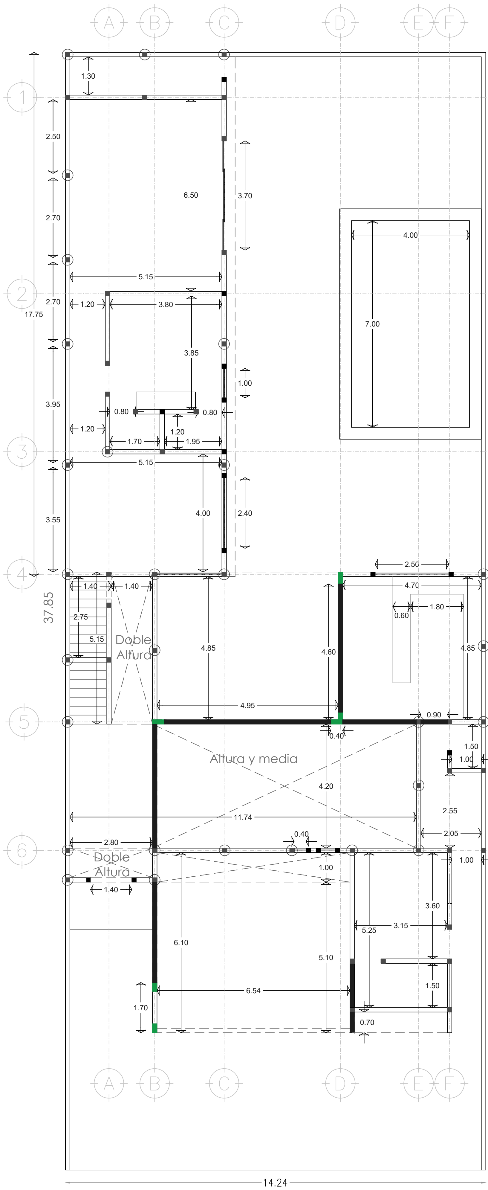
PLANTA BAJA
