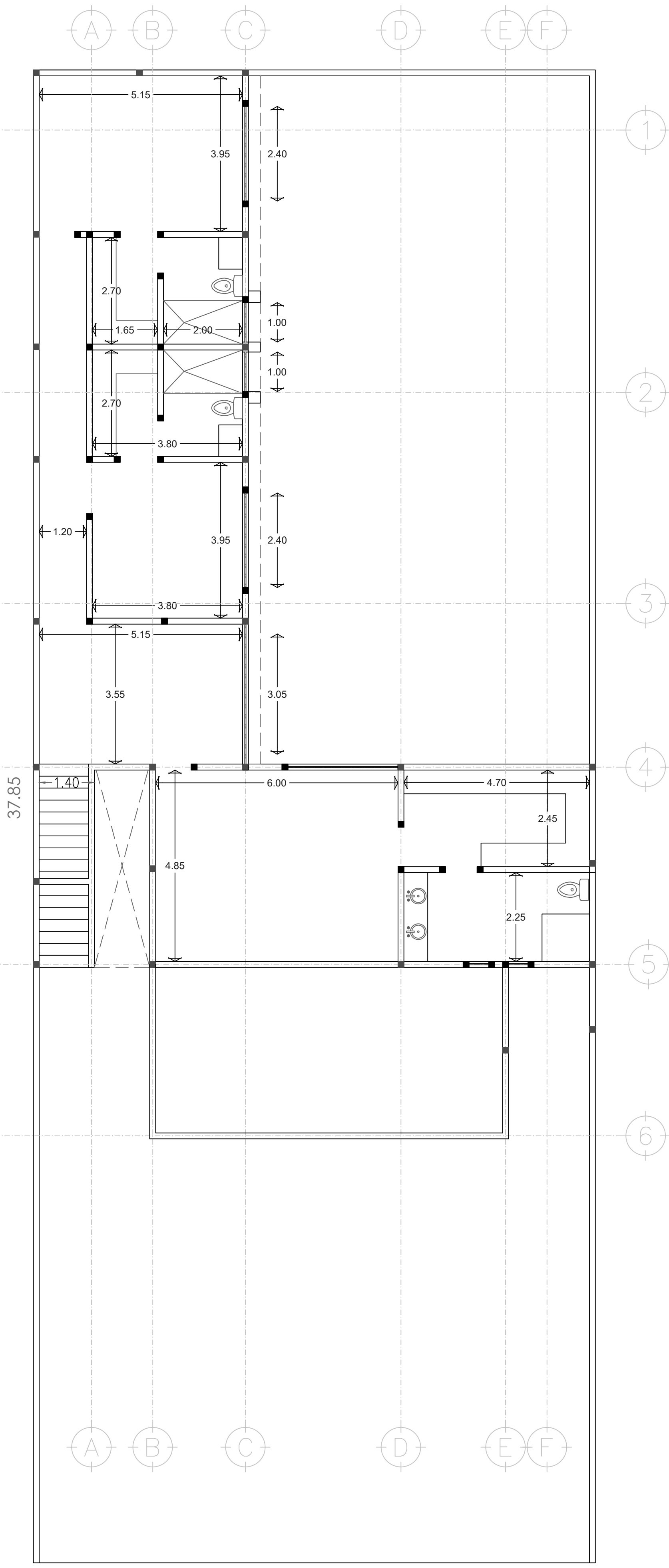
PLANTA ALTA
