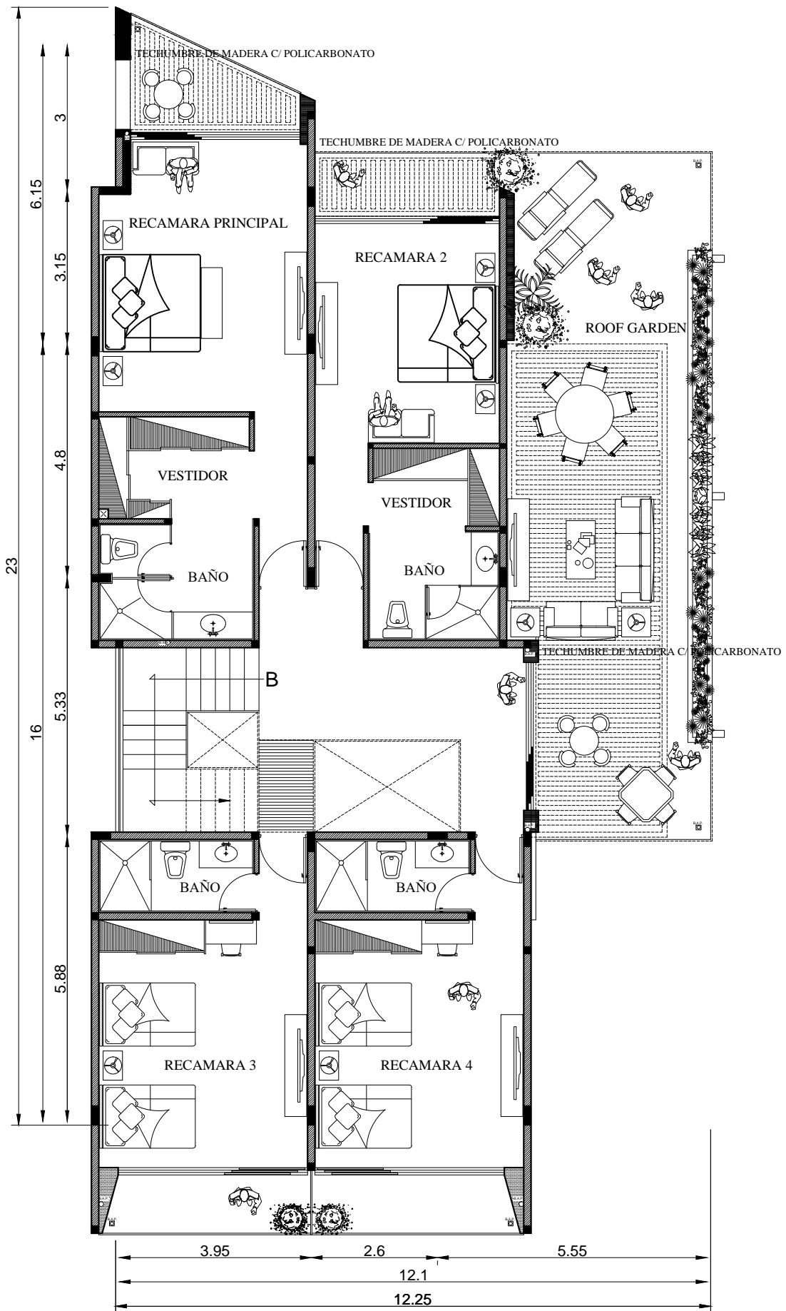
ARQ. PLANTA ALTA VILLA 1 - 6
