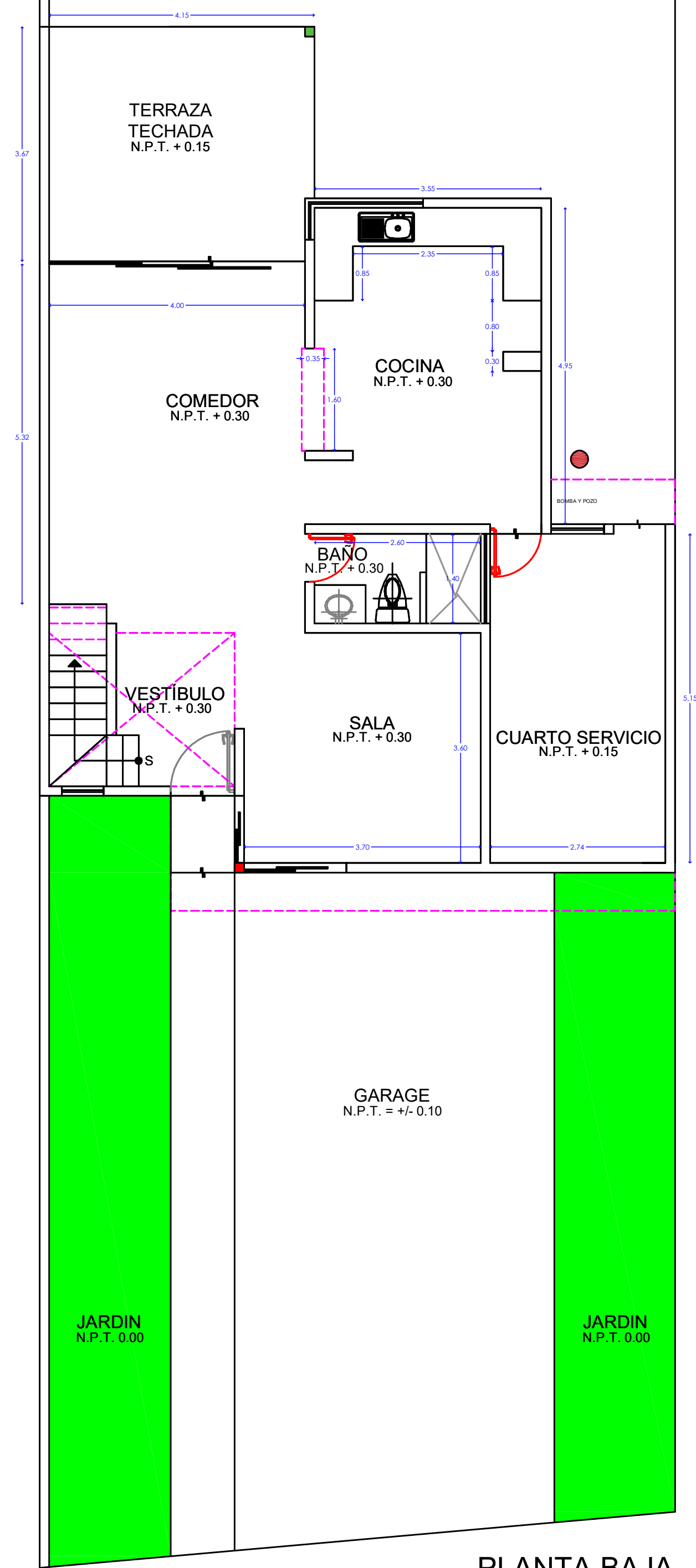
PLANTA BAJA
