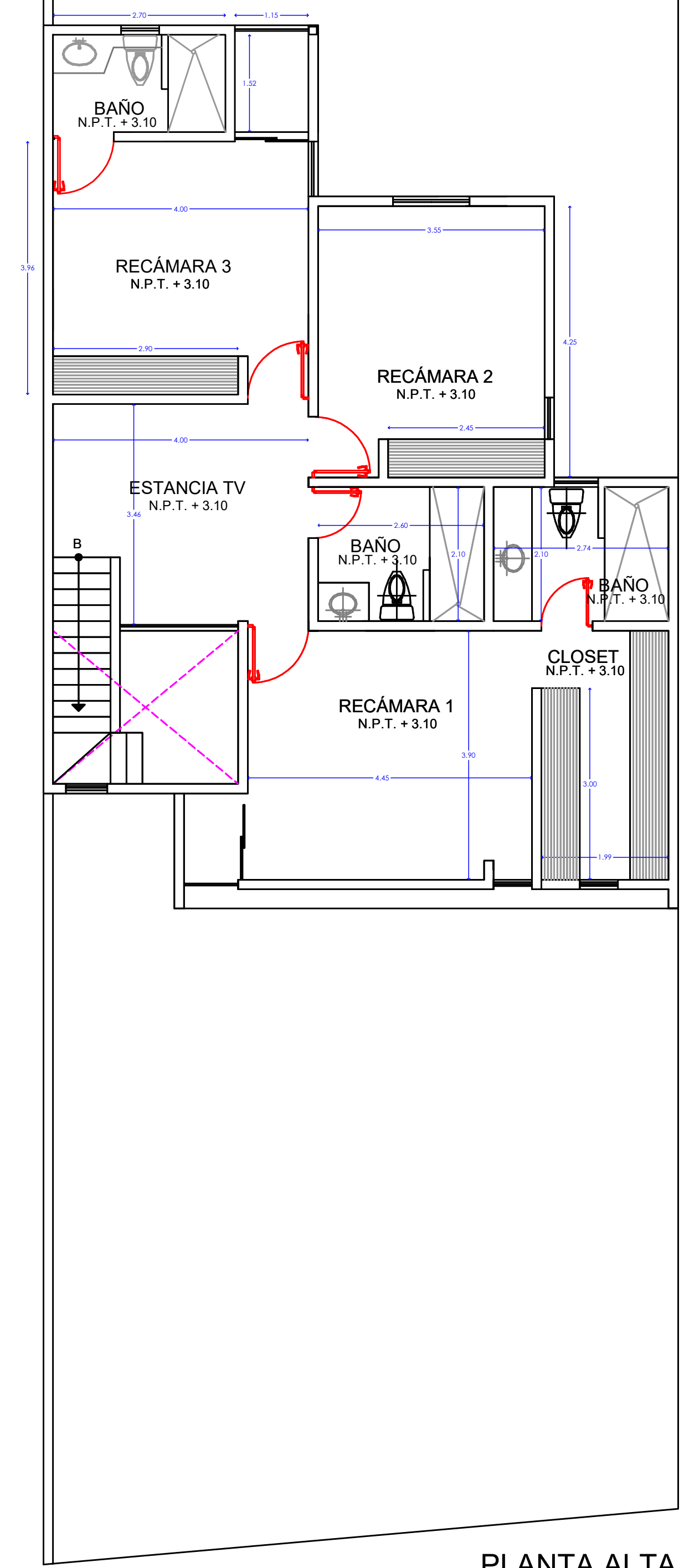
PLANTA ALTA
