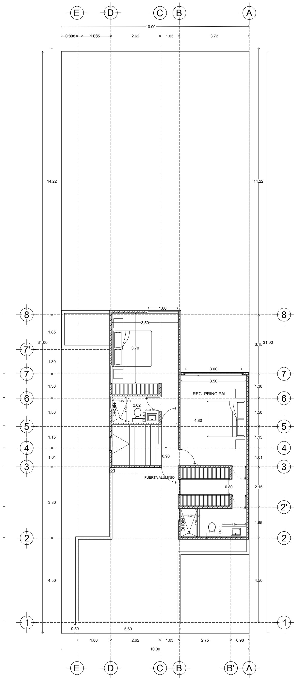
PLANTA ALTA
