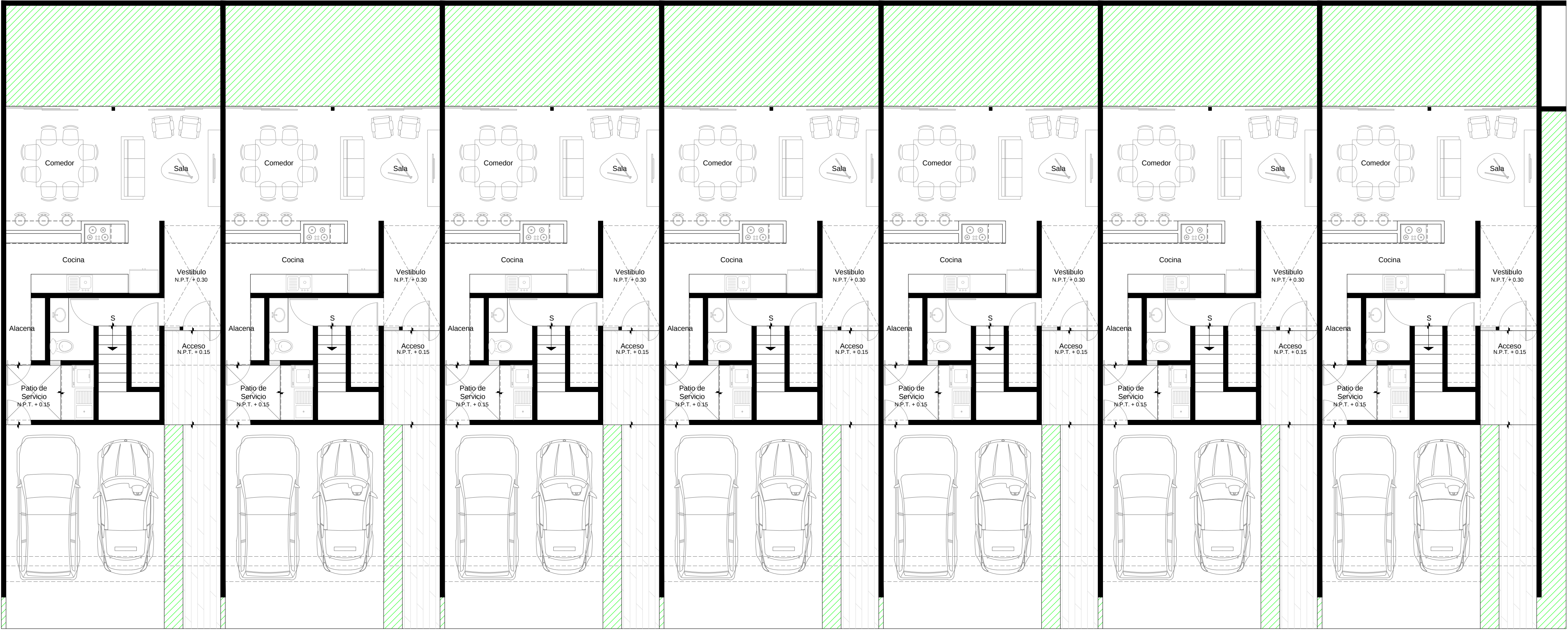
Planta Baja
