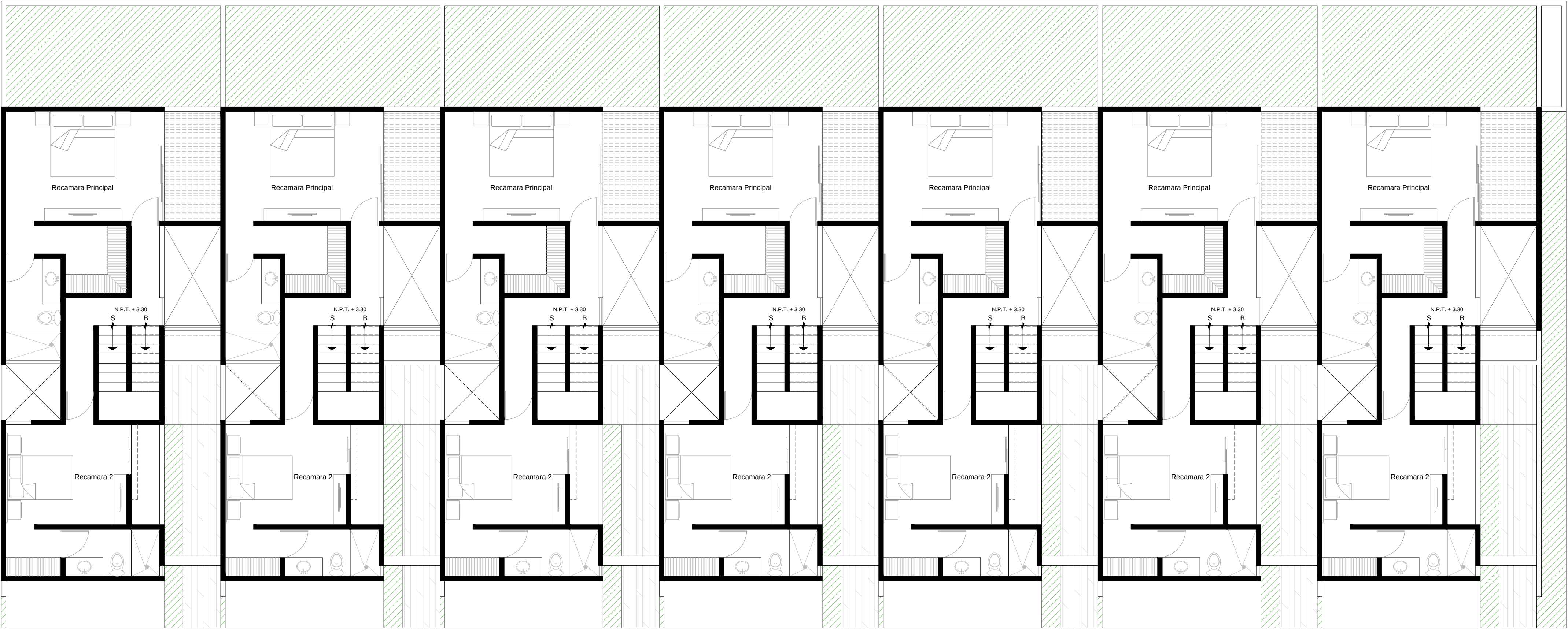
Planta Nivel 1
