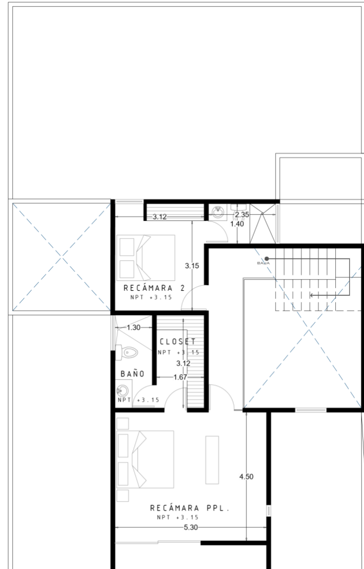
PLANTA ALTA
