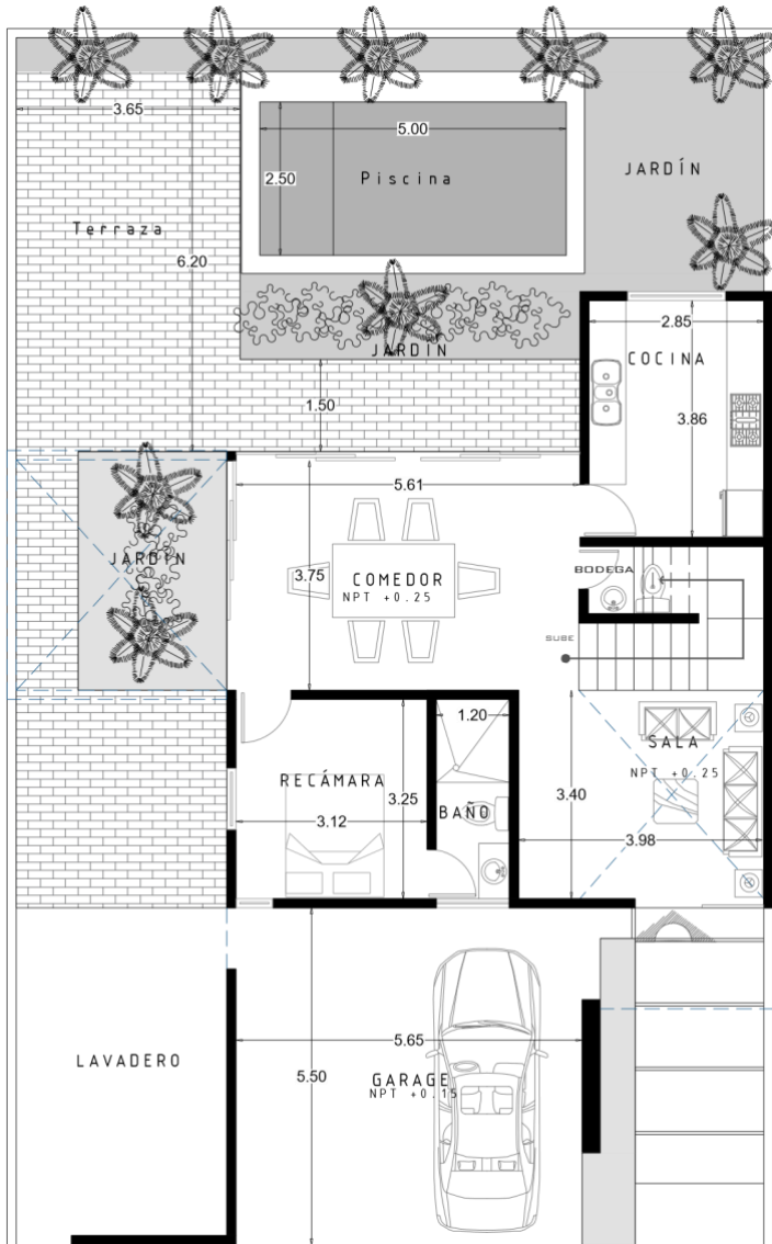
PLANTA
