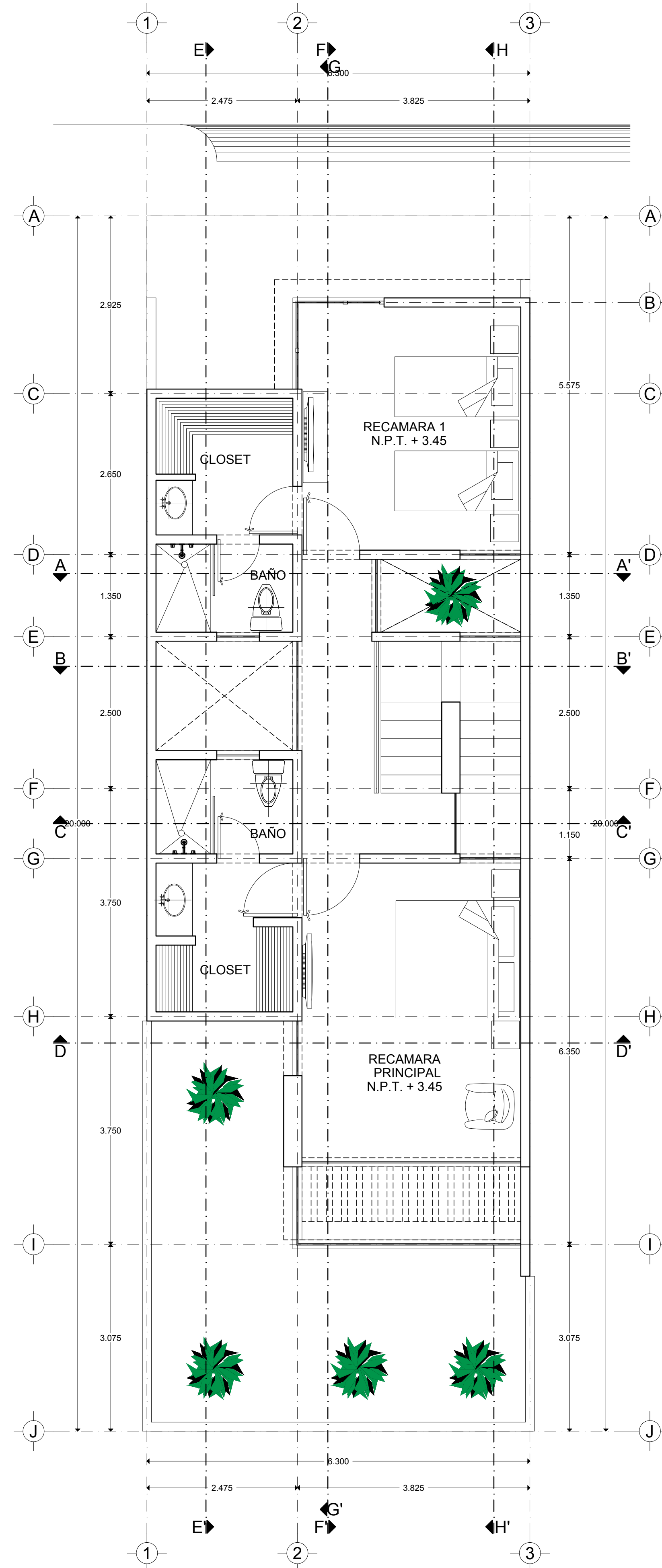
PLANTA PRIMER NIVEL
