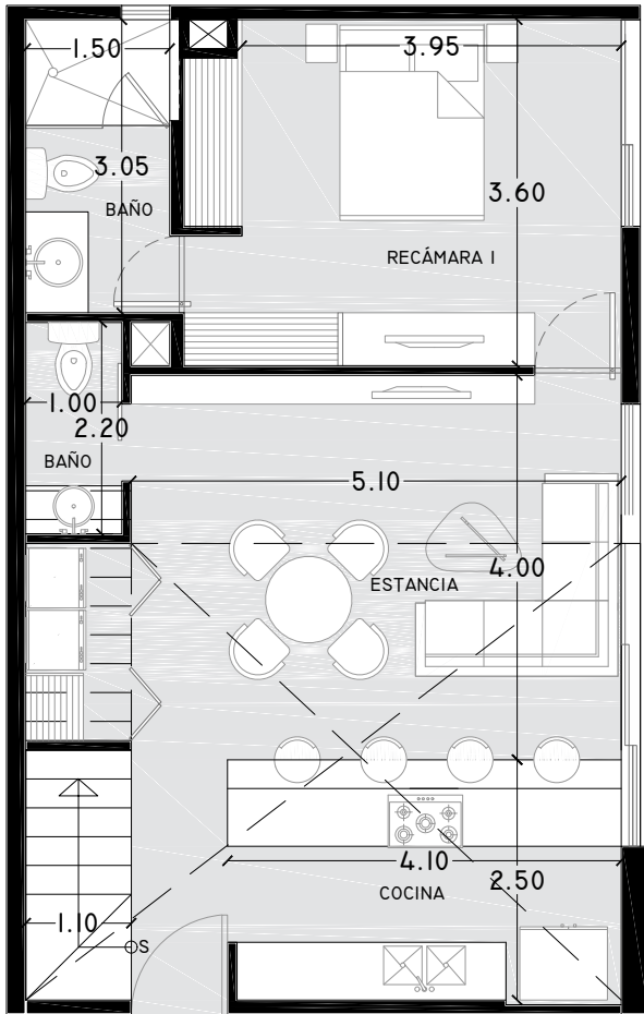
PLANTA BAJA DEPTO STUDIO
