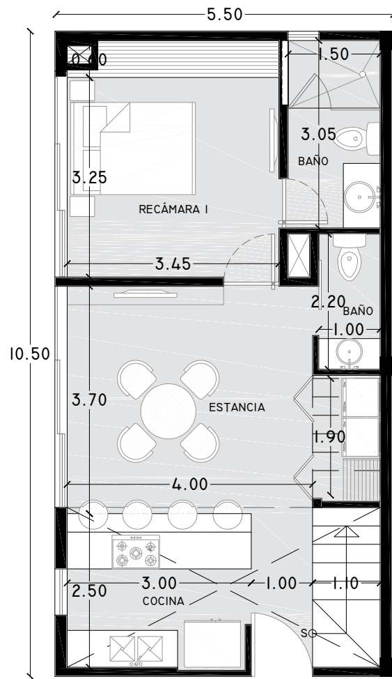
PLANTA BAJA DEPTO STUDIO
