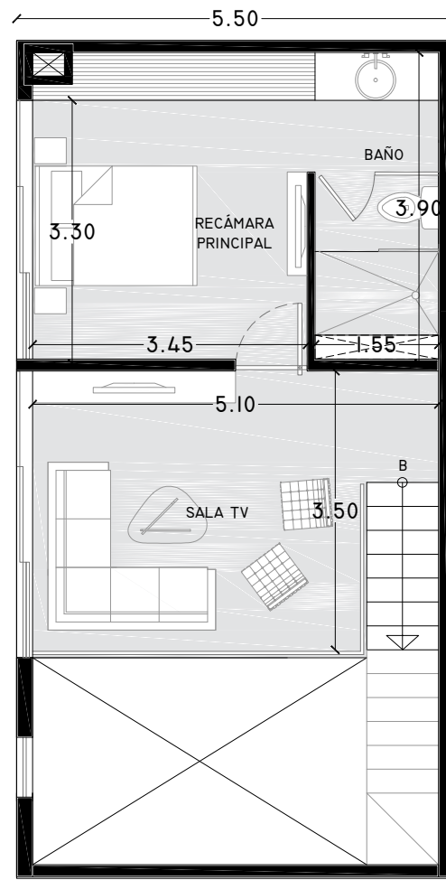
PLANTA ALTA DEPTO STUDIO
