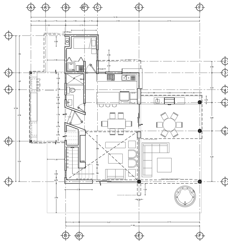
PLANTA BAJA
