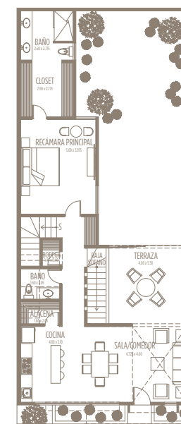
PLANTA BAJA
