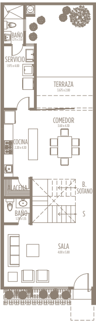
PLANTA BAJA
