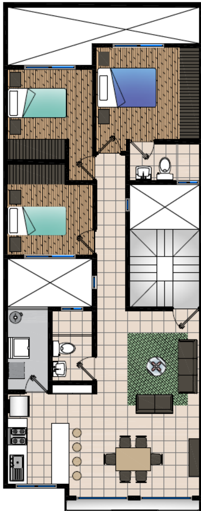
PLANTA TIPO DEPARTAMENTO
