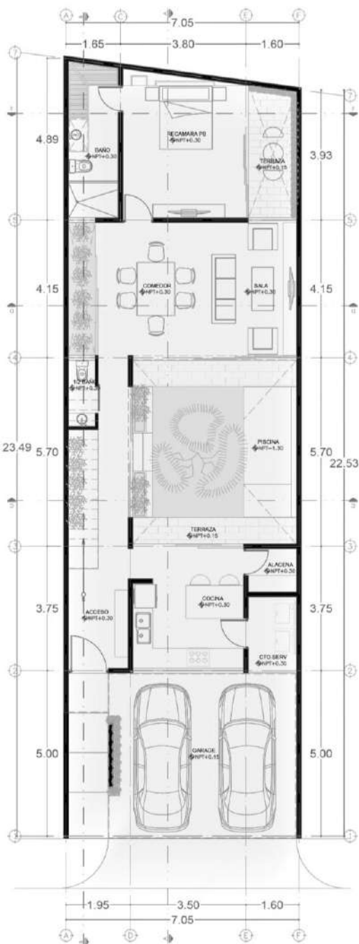
PLANTA BAJA
