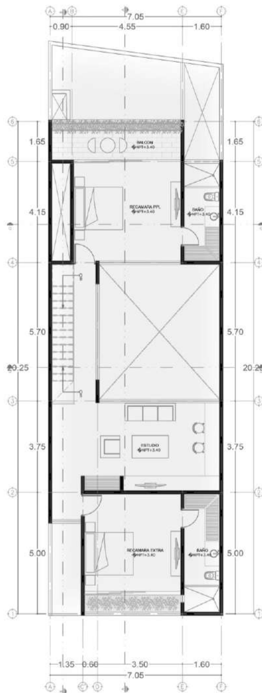
PLANTA ALTA
