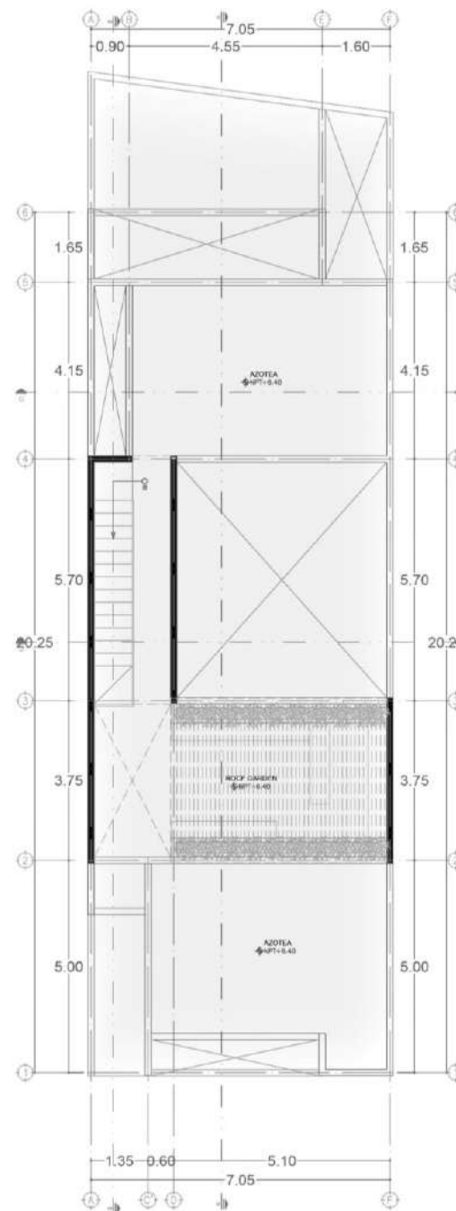
PLANTA AZOTEAS
