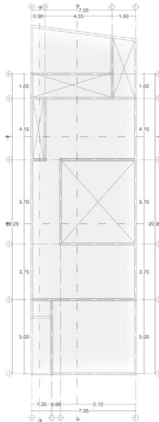
PLANTA AZOTEAS
