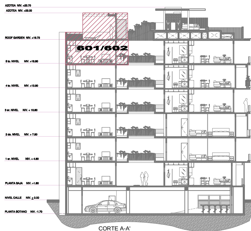
UBICACIÓN DEPARTAMENTOS 601 Y 602 EN ALZADO
