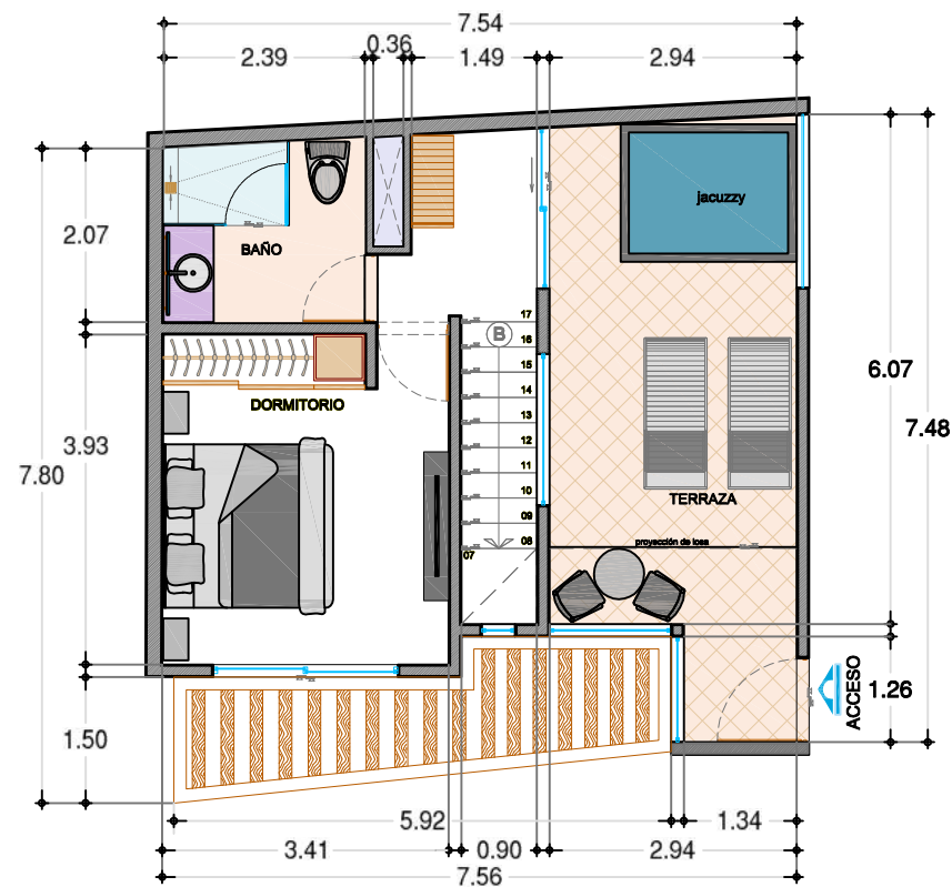
DEPARTAMENTOS "601 Y 602" PLANTA ALTA ARQUITECTONICA
