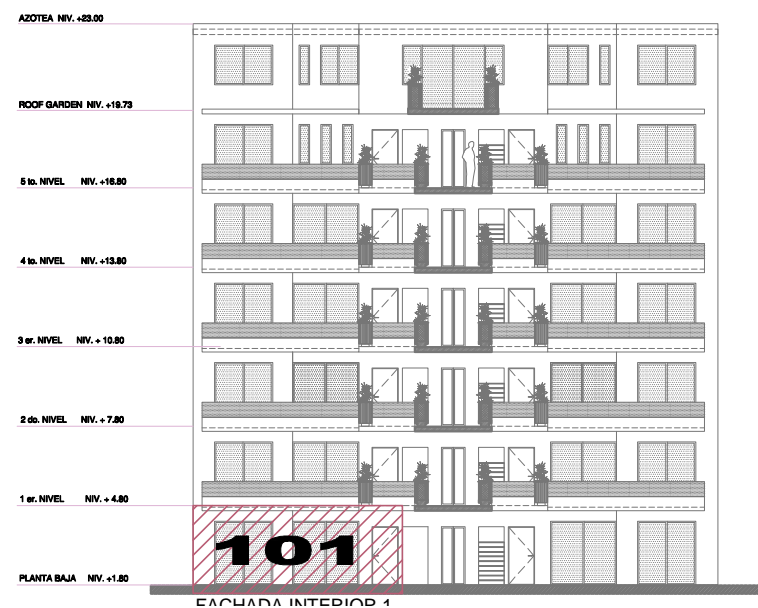
UBICACIÓN DEPARTAMENTOS 101 EN ALZADO
