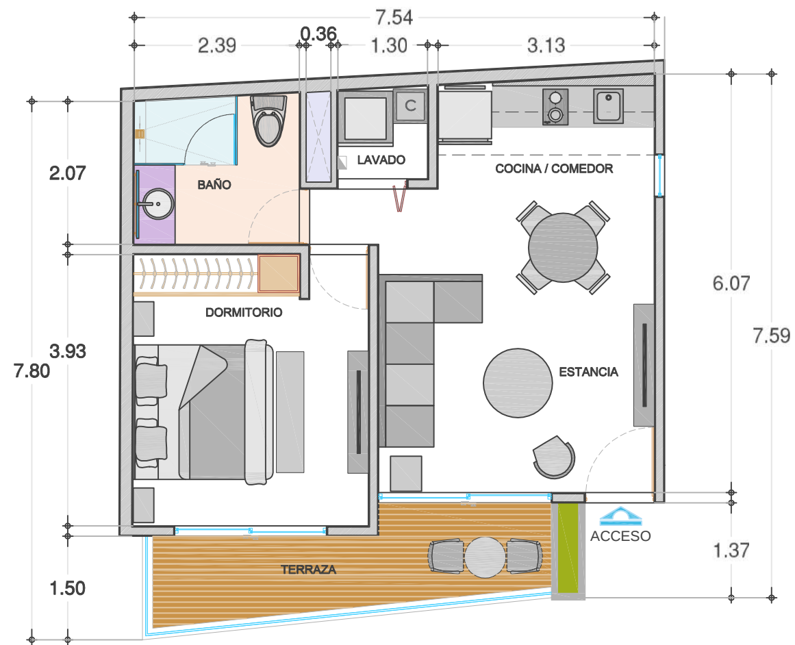
DEPARTAMENTOS "201,202, 301, 302, 401, 402, 501,502" PLANTA ARQUITECTONICA
