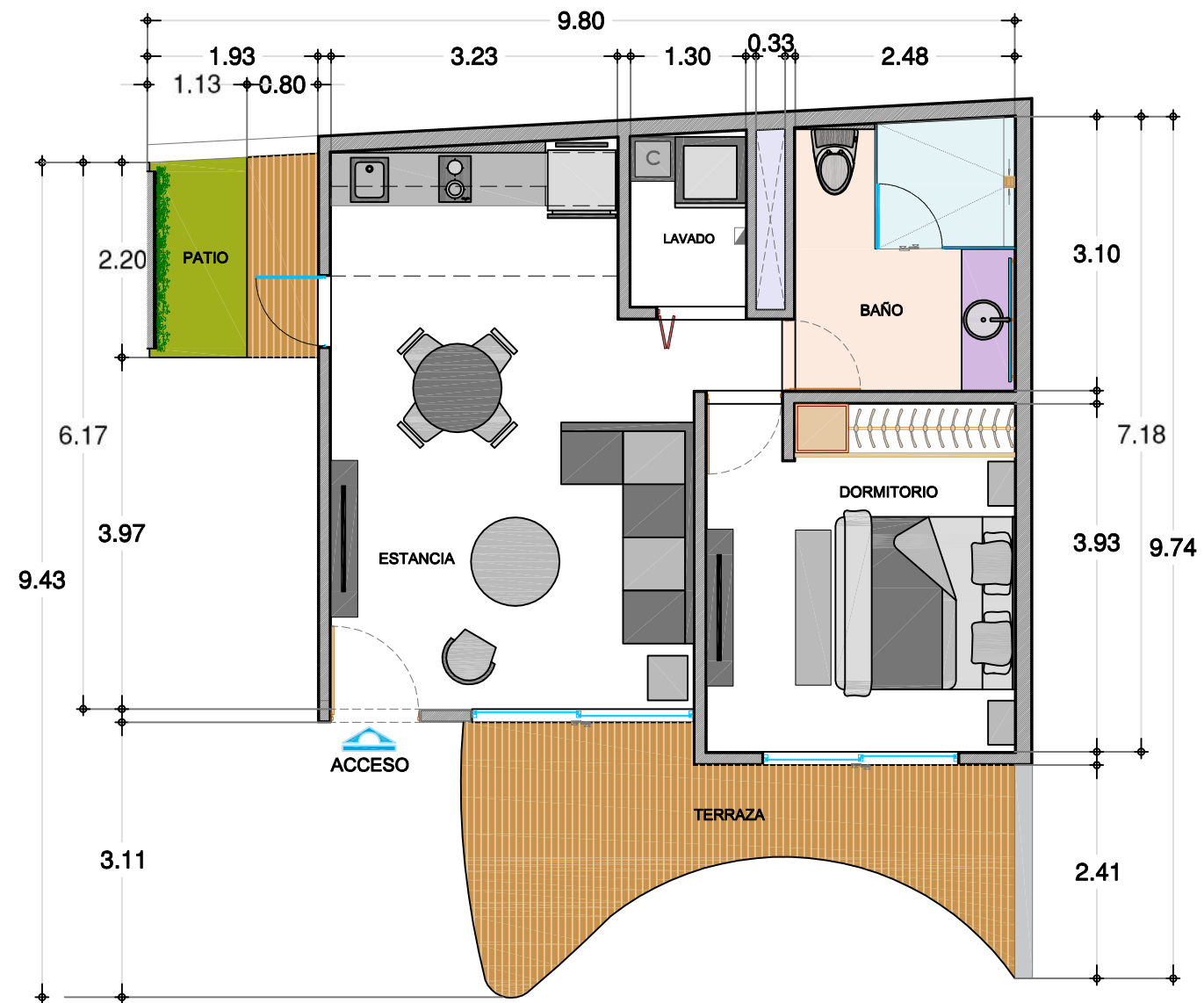
DEPARTAMENTO "102 " PLANTA ARQUITECTONICA
