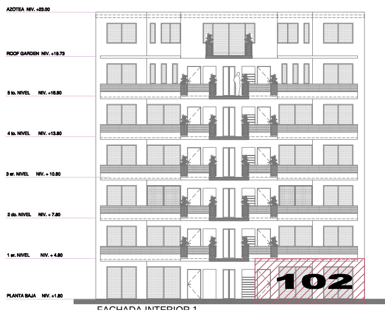
UBICACIÓN EN PLANTA DEPARTAMENTO 102
