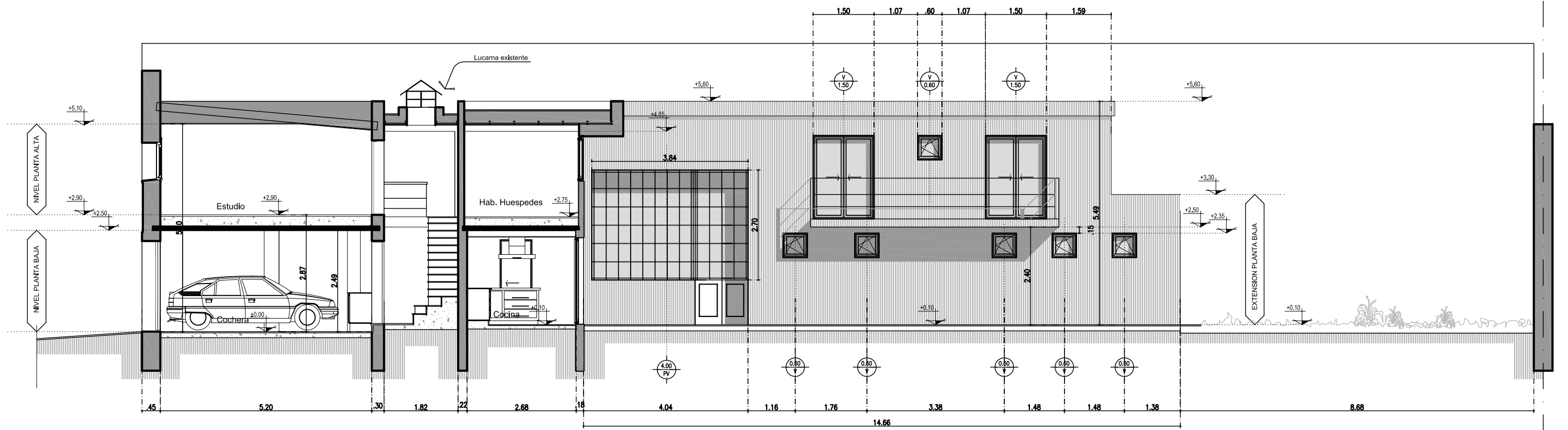
CORTE A-A + FACHADA ESC.: 1:50
