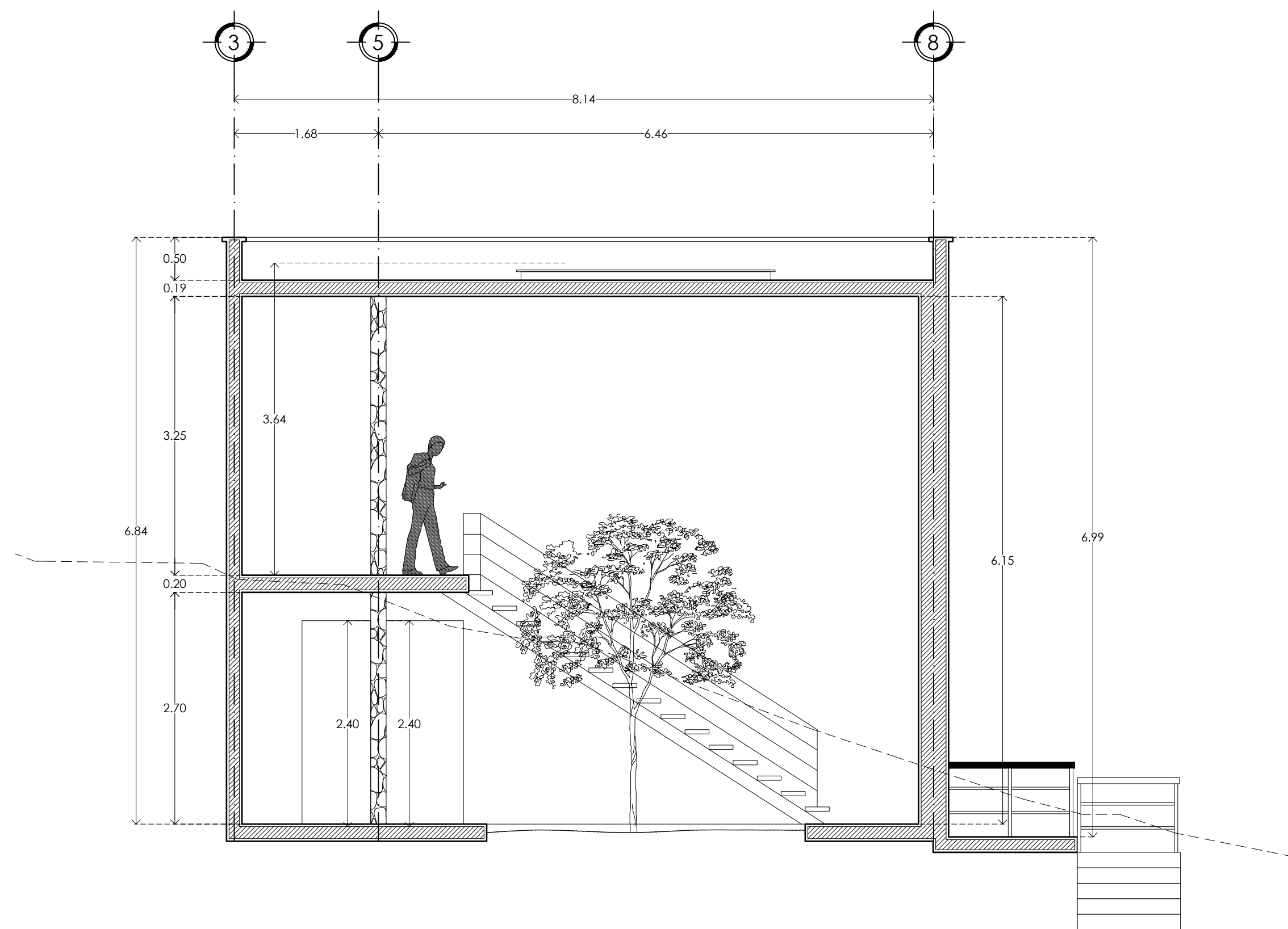
SECCIÓN B-B
