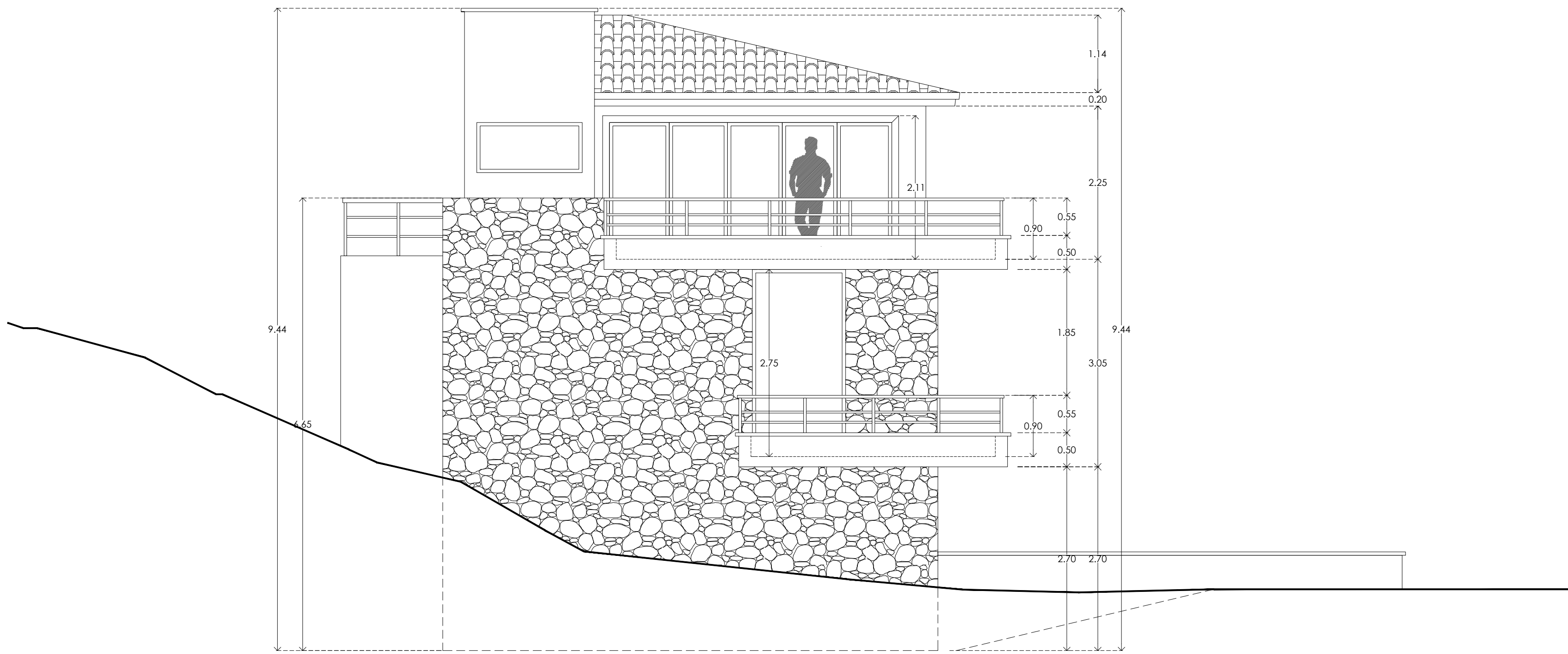
FACHADA LATERAL ESC. 1:100
