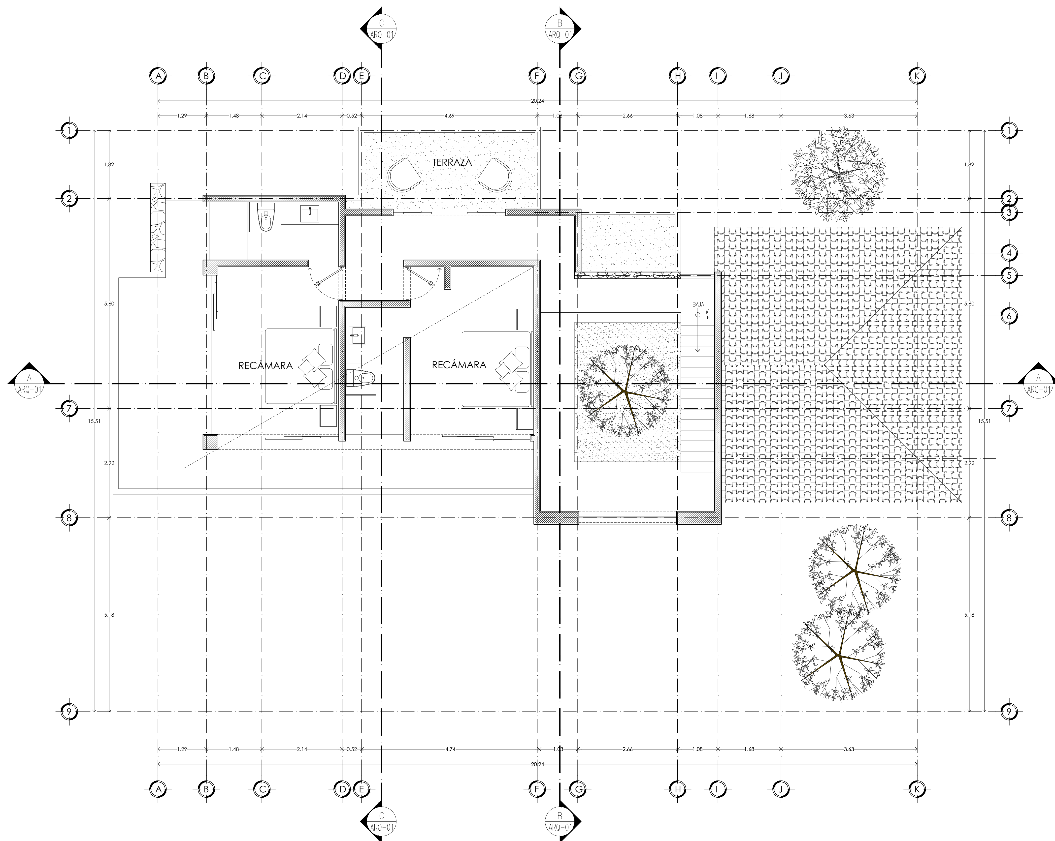
PLANTA ALTA
