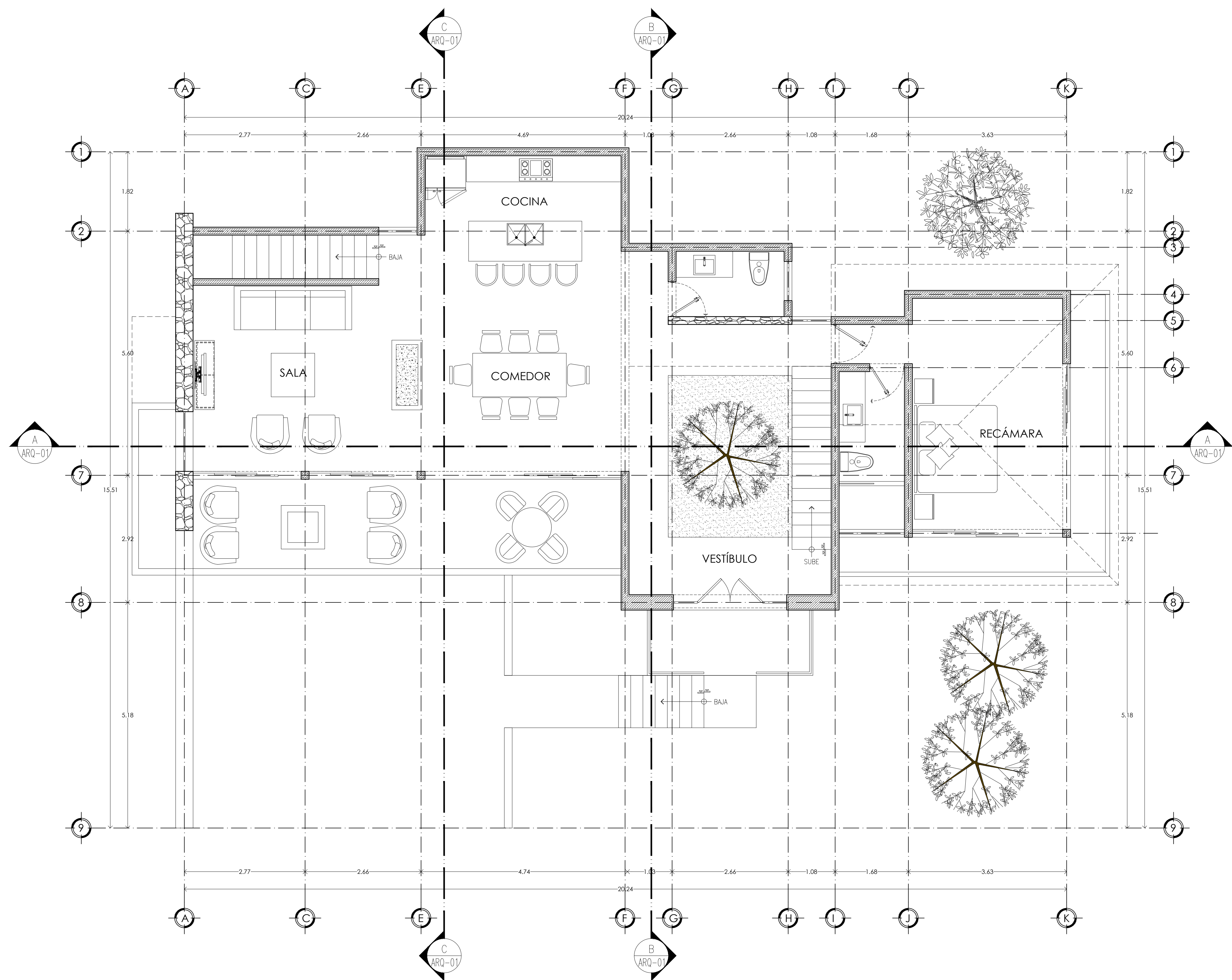
PLANTA BAJA ESC. 1:50
