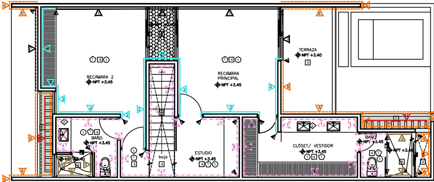
PLANTA ALTA
