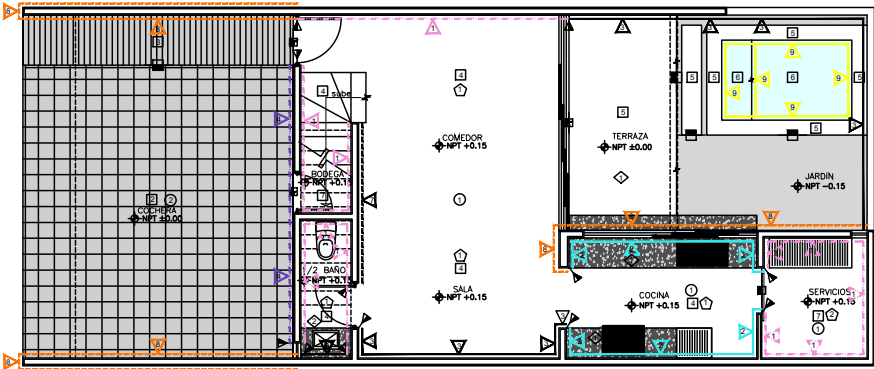
PLANTA BAJA
