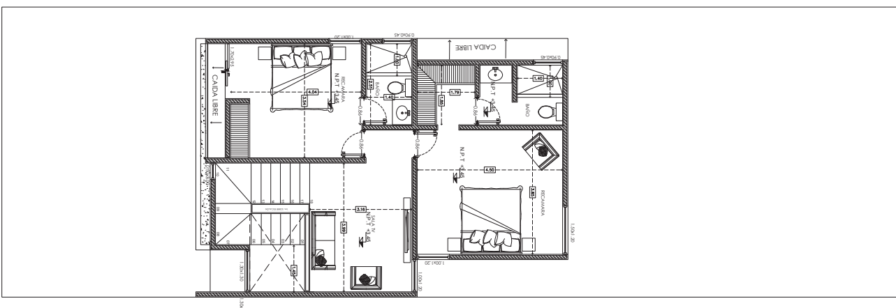
Planta alta
