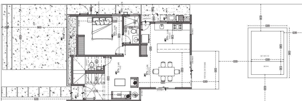
Planta baja
