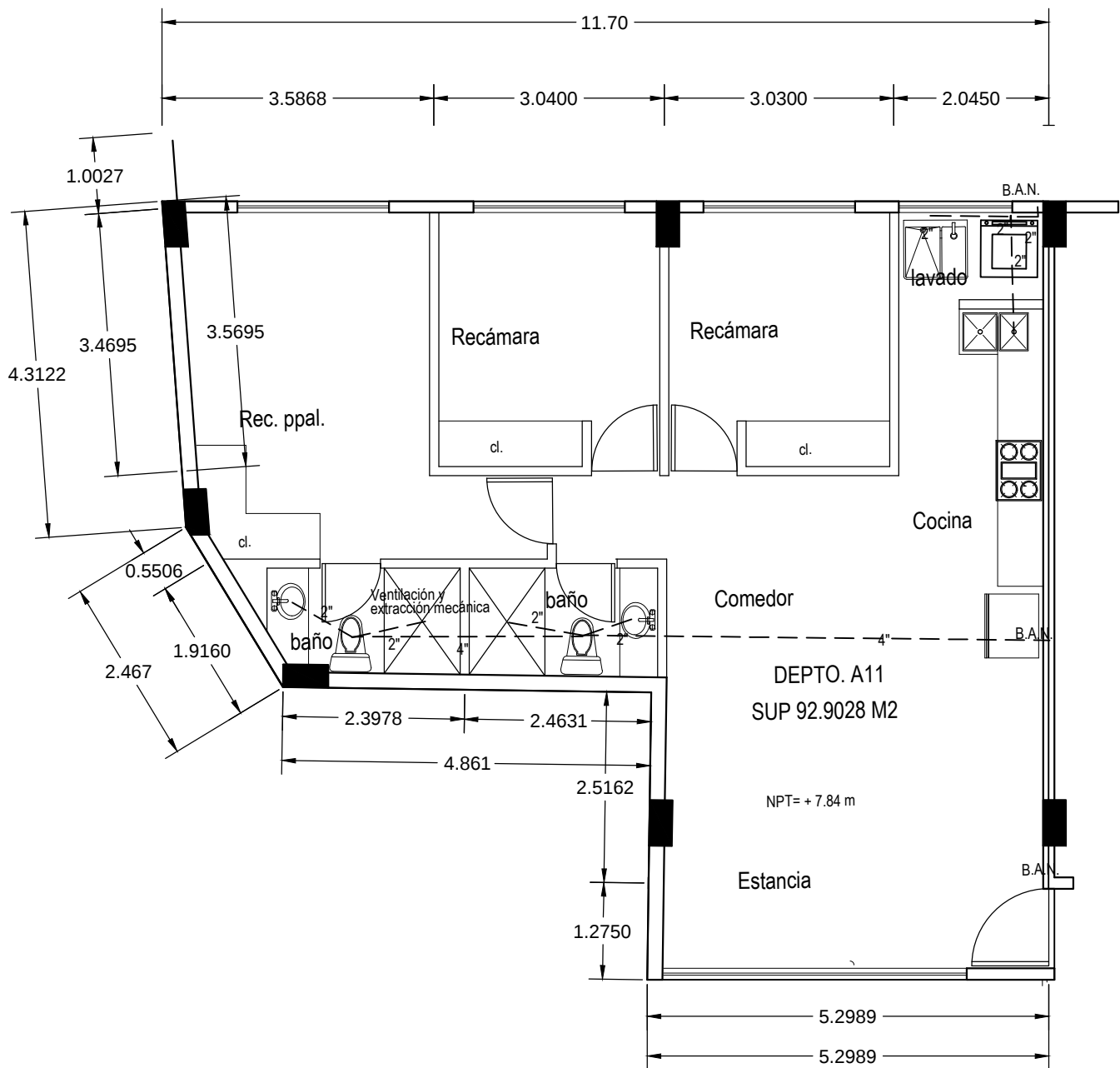
PLANTA ARQUITECTONICA DEPTO A11 SUP 92.9028 M2
