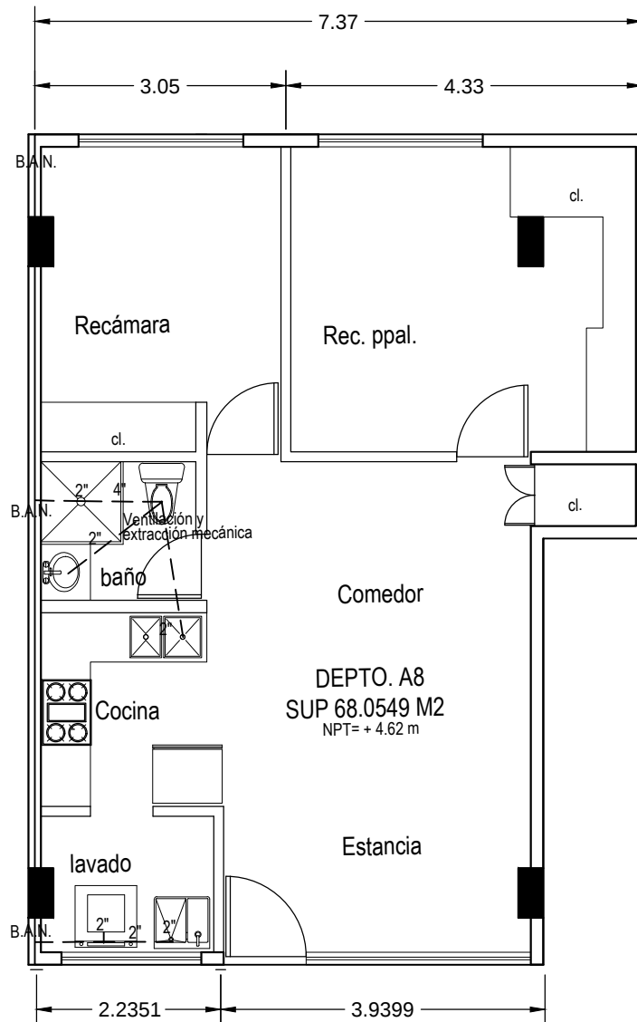
PLANTA ARQUITECTONICA DEPTO A8 SUP 68.0549 M2
