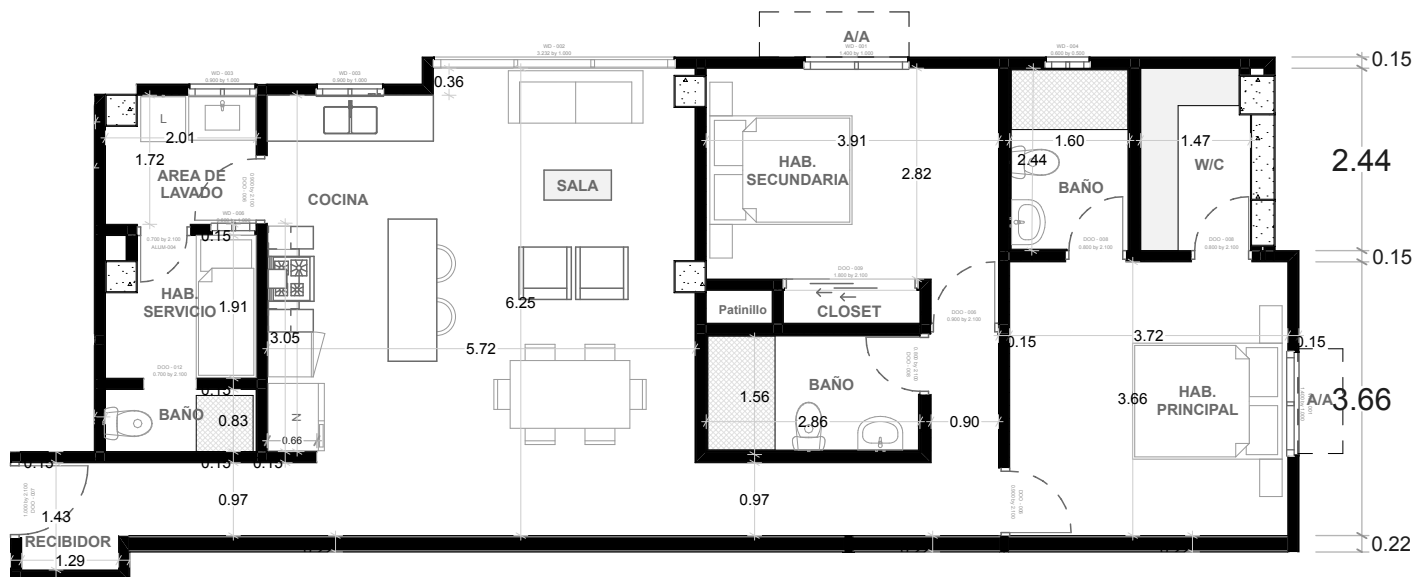
1 Planta Arquitectónica TIPO C 1:100
