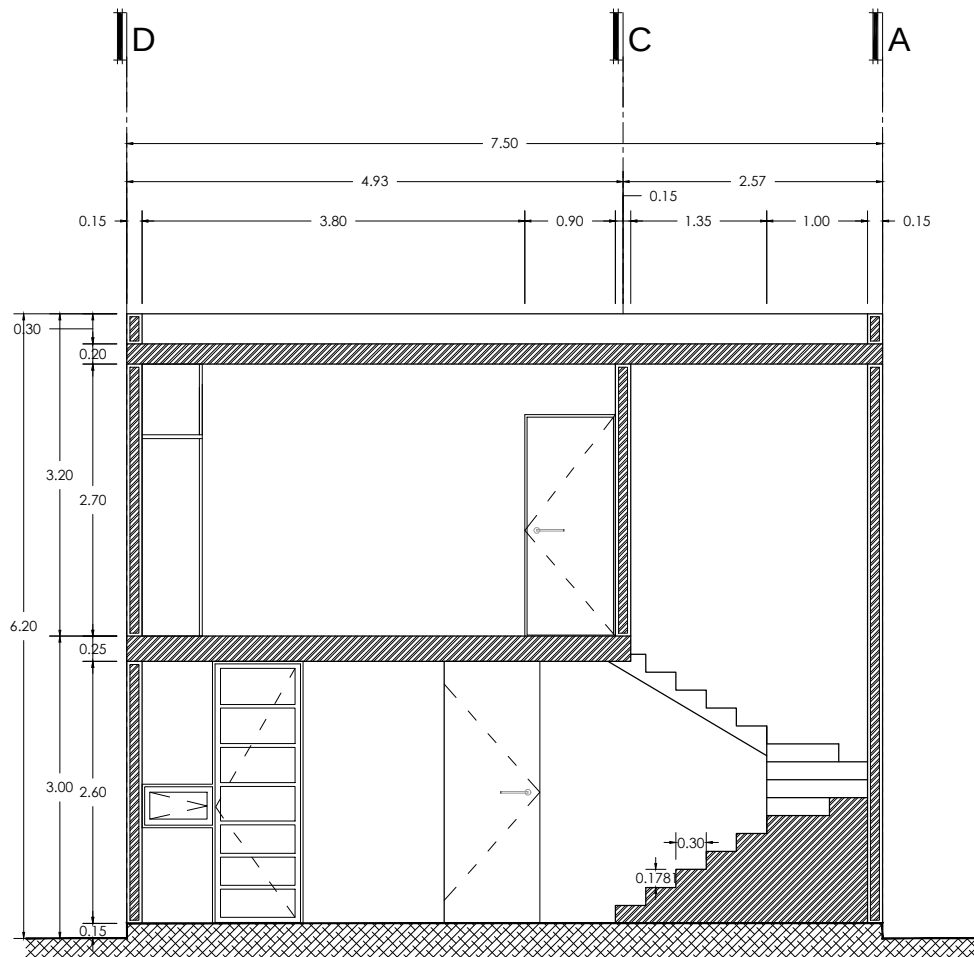
Corte Transversal B-B'
