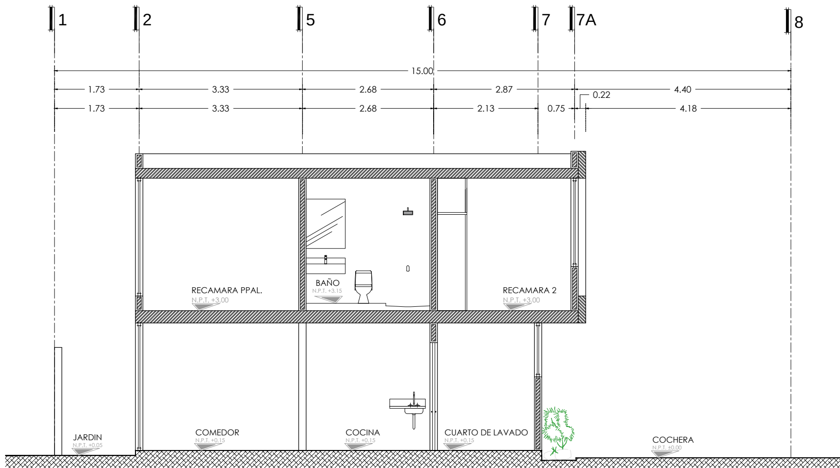
Corte Longitudinal A-A'
