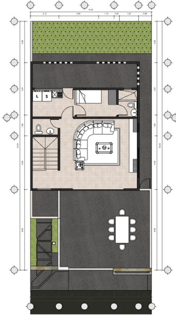
NIVEL 2
