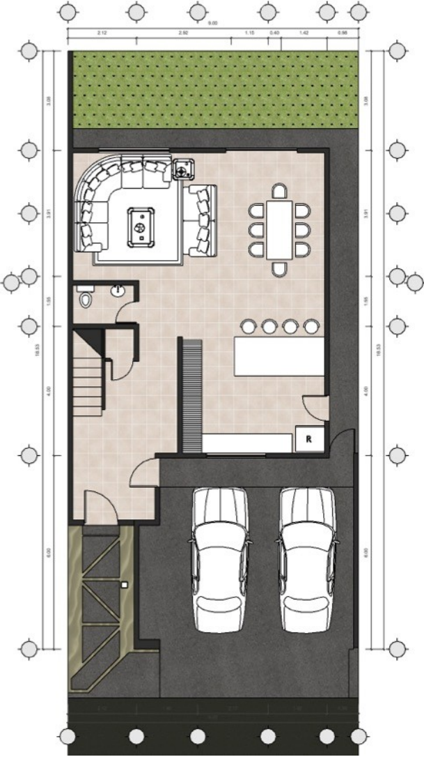
PLANTA BAJA
