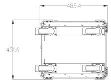
Bottom
