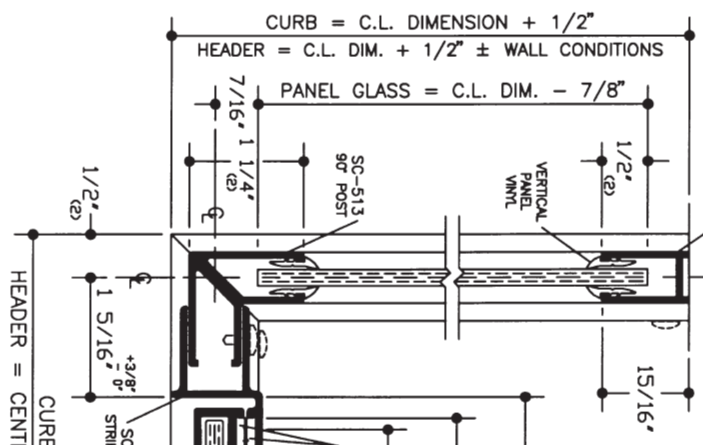
FRAMELESS DOOR PANEL
