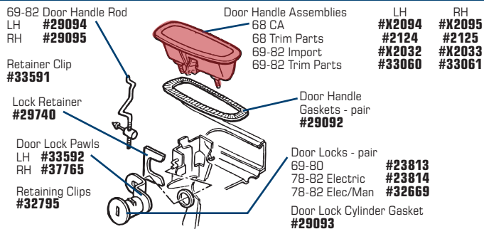
#X2032 1969-82 Door Handle Assembly - LH
