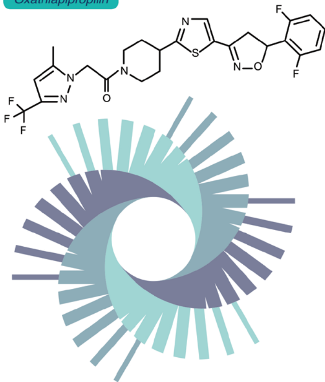
Oxathiapropilin
